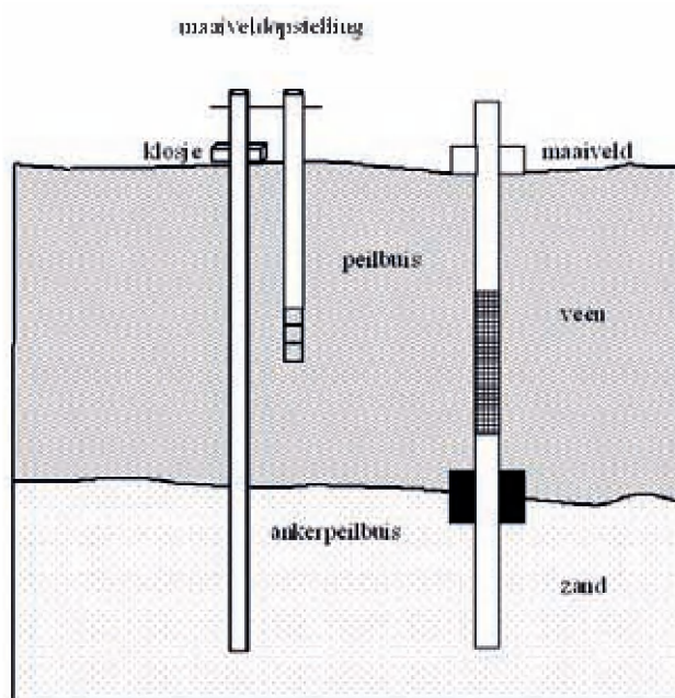
FIGUUR 3.7 MAAVELDOPSTELLING VOLGENS HET PEILBUIS-ANKERBUIS PRINCIPE (LINKS) EN PEILBUIS VERANKERD IN ZANDONDERGROND (RECHTS) (BRON: STAATSBOSBEHEER, 2000 EN GROBBE, T., WATERSCHAP VELD EN VECHT)
