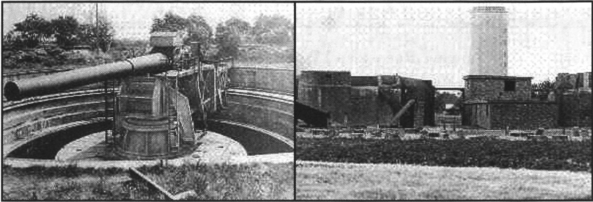
Eerste wereldoorlog batterij Deutschland
