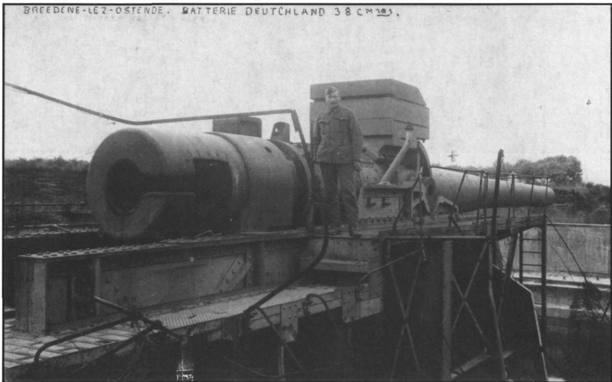
AFB. 13. IN SEPTEMBER 1915 WORDT OP DE GRENS TUSSEN BREDENE EN KLEMSKERKE GESTART MET DE BOUW VAN ' BATTERIJ DEUTSCHLAND ', OOK WEL ' BATTERIJ JACOBINESSEN ' GENAAMD NAAR DE DICHTBIJ GELEGEN HOEVE. DE VIER 38 CM KANONNEN HADDEN EEN SCHOOTSAFSTAND VAN MEER DAN 40 KM EN REIKTEN DAARMEE VAN DUINKERKE TOT AAN HET EILAND WALCHEREN. OM HET EMPLACEMENT TE BEDIENEN WERD SPECIAAL VANUIT OOSTENDE, OVER BREDENE-AAN-ZEE, EEN SPOORLIJN AANGELEGD.
