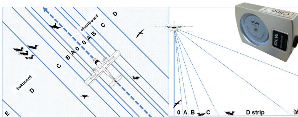
Figuur 2.2 Schematische weergave van waarneemstrips vanuit een vliegtuig in bovenaanzicht (links) en vooraanzicht (rechts). De hoeken behorende bij stripgrenzen zijn zogeheten 'clinohoeken' (zie tabel 2.1) en worden gemeten met een clinometer (inzet). Schematic representation of strip transects from the survey plane in top view (left) and front view (right). Angles of strip boundaries (see table 2.1) are measured with a clinometer (inset).
