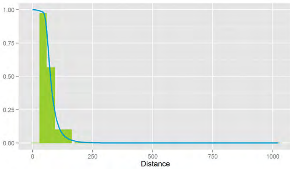
Figuur III.15a&b Distance detectiecurve voor zeeoet (Hazard Rate). Distance detection curve of Common Guillemot (Hazard Rate).
