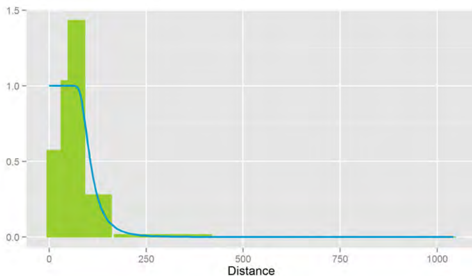
Figuur III.1 Distance detectiecurve voor roodkeelduiker (Hazard Rate) zonder left-truncation omdat deze soort met name opvliegt en niet onderduikt in de waarnemingsstrips onder het vliegtuig. Distance detection curve of Red-throated Diver (Hazard Rate) without left-truncation because this species primarily flies instead of dives in the most inner observation bands in response to the survey plane.
