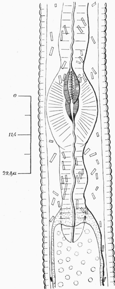
Fig. 11. — Walcherenia typica . Eindbulbus van den slokdarm van een vrouwtje, met fijnere, innerlijke structuur, en Cardia.
