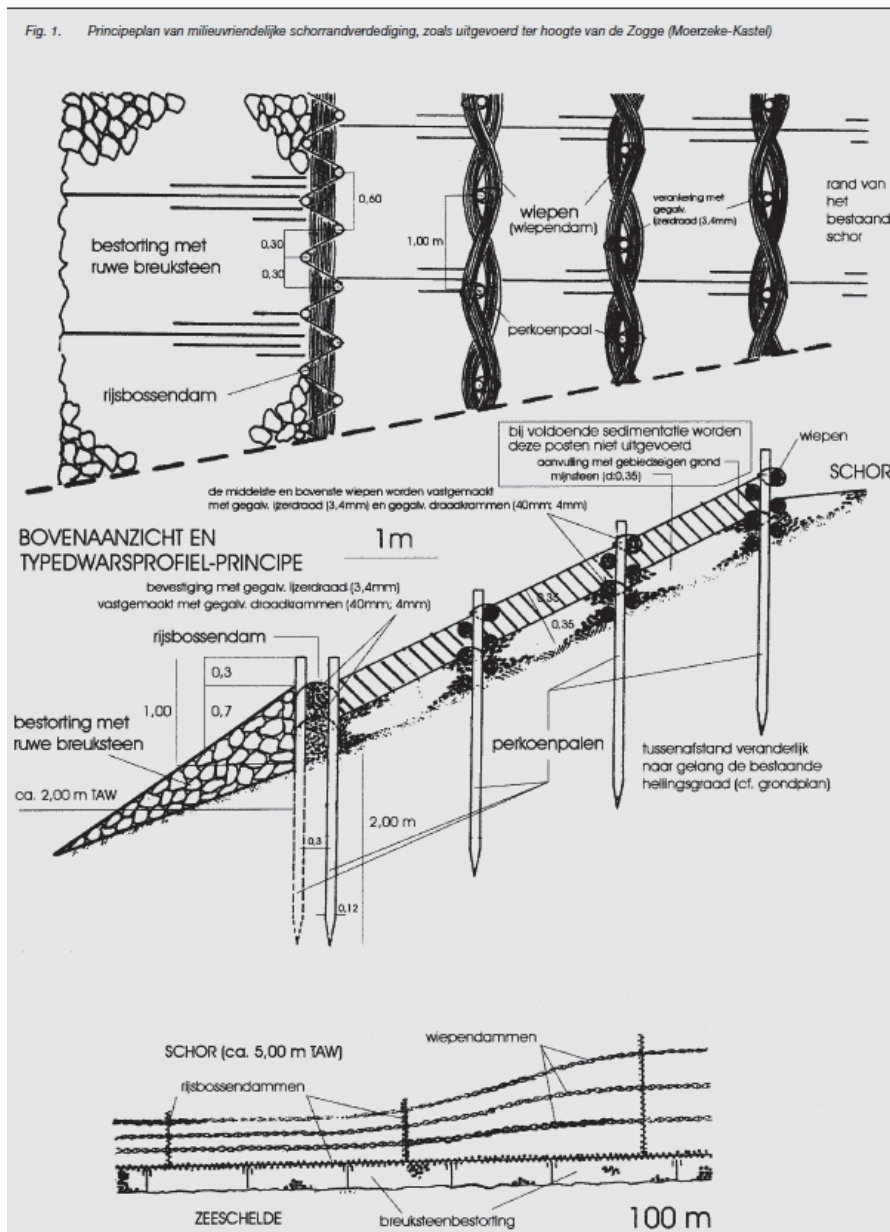
Figuur 2-7: schorrandverdediging op basis perkoenpalen met daartussen gevlochten wiepen (Hoffmann & Meire, 1997).
