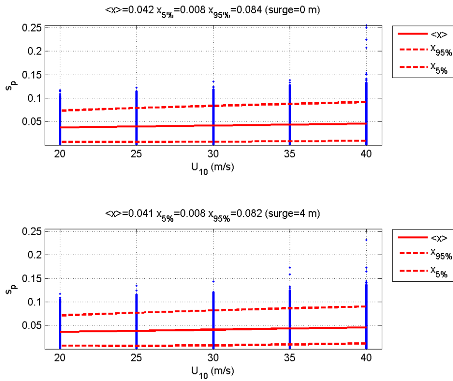
Figuur 4.30 s_p vs U_{10} SWAN resultaten voor de Westerschelde voor offshore waterstanden van 4 m+NAP (grafiek boven) en 0 m+NAP (grafiek beneden).
