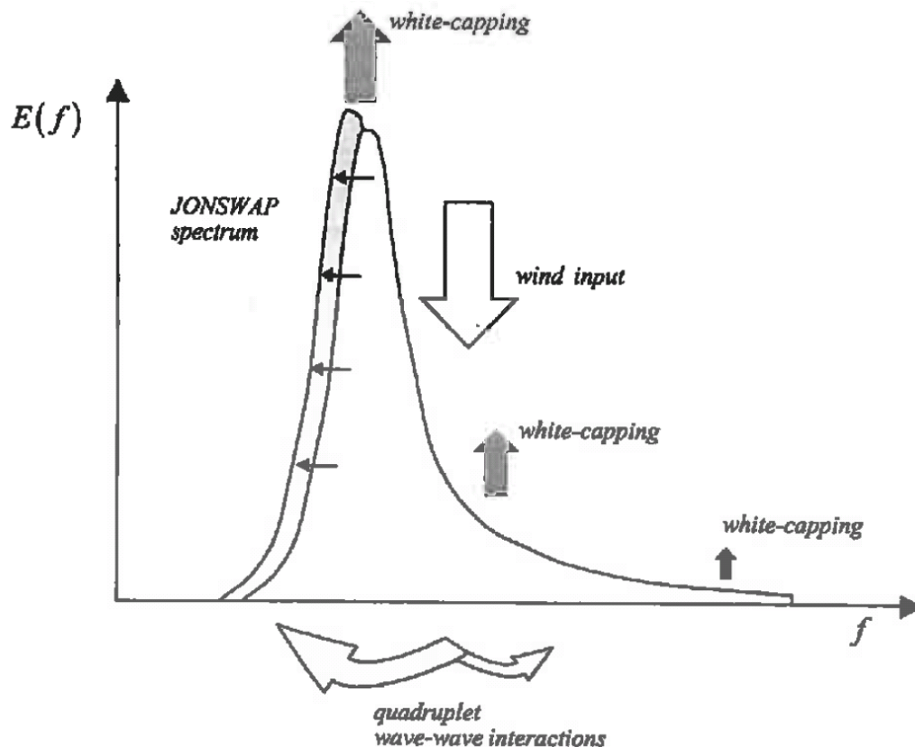
Figuur 2.2 Schematisatie van de golfspectrale vervorming door de diepwater golfenergie brontermen. Bron: Grafiek uit Holthuisen (2007, Figuur 6.27).
