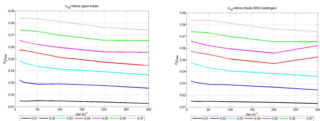
Figuur 4.1 (s_p)_{\max} vs de bodemhelling. De kleur van de lijnen geeft de waarde van s_{ep} op diep water. Figuur links: SWAN simulaties met 40 m/s windsnelheid en geen triads. Figuur rechts: SWAN simulaties met 40 m/s windsnelheid en triads conform de instellingen zoals voorbereid binnen SBW.
