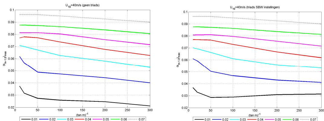
Figuur 4.2 (s_{m-1,0})_{max} vs de bodemhelling. De kleur van de lijnen geeft de waarde van s_{op} op diep water. Figuur links: SWAN simulaties met 40 m/s windsnelheid en geen triads. Figuur rechts: SWAN simulaties met 40 m/s windsnelheid en triads conform de in SBW afgeleide instellingen.
