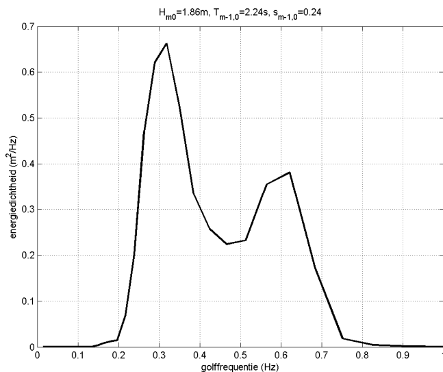
Figuur 4.32 Voorbeeld van een SWAN spectrum voor de Westerschelde met een extreem hoge golfsteilheid, s_{m-1,0} = 0.24 . Dit spectrum is geassocieerd met een windsnelheid van 35 m/s en een richting van 300°N in de SWAN berekeningen en de locatie (274, zie Figuur 2.7) is dichtbij WAL5 in Figuur 2.9.
