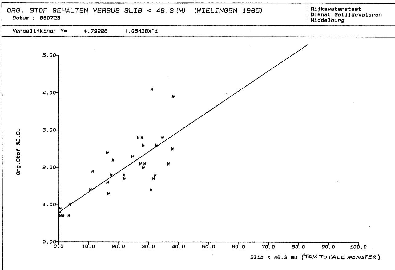
Figuur 6 - Organische stof gehalten (% D.S.) versus slib < 48.3 μm (t.o.v. totale monster) a.d.h.v. 32 "de Spleet" bodemonsters (M).
