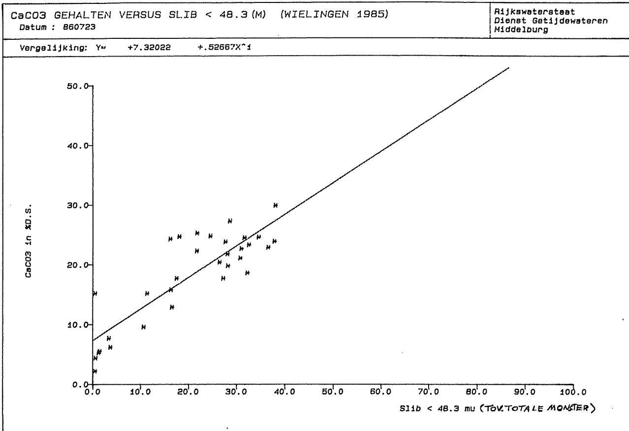
Figuur 5. CaCO 3 gehalten (% D.S.) versus slib 48.3 μm (t.o.v. totale monster) a.d.h.v. 32 "de Spleet" bodemonsters (M).
