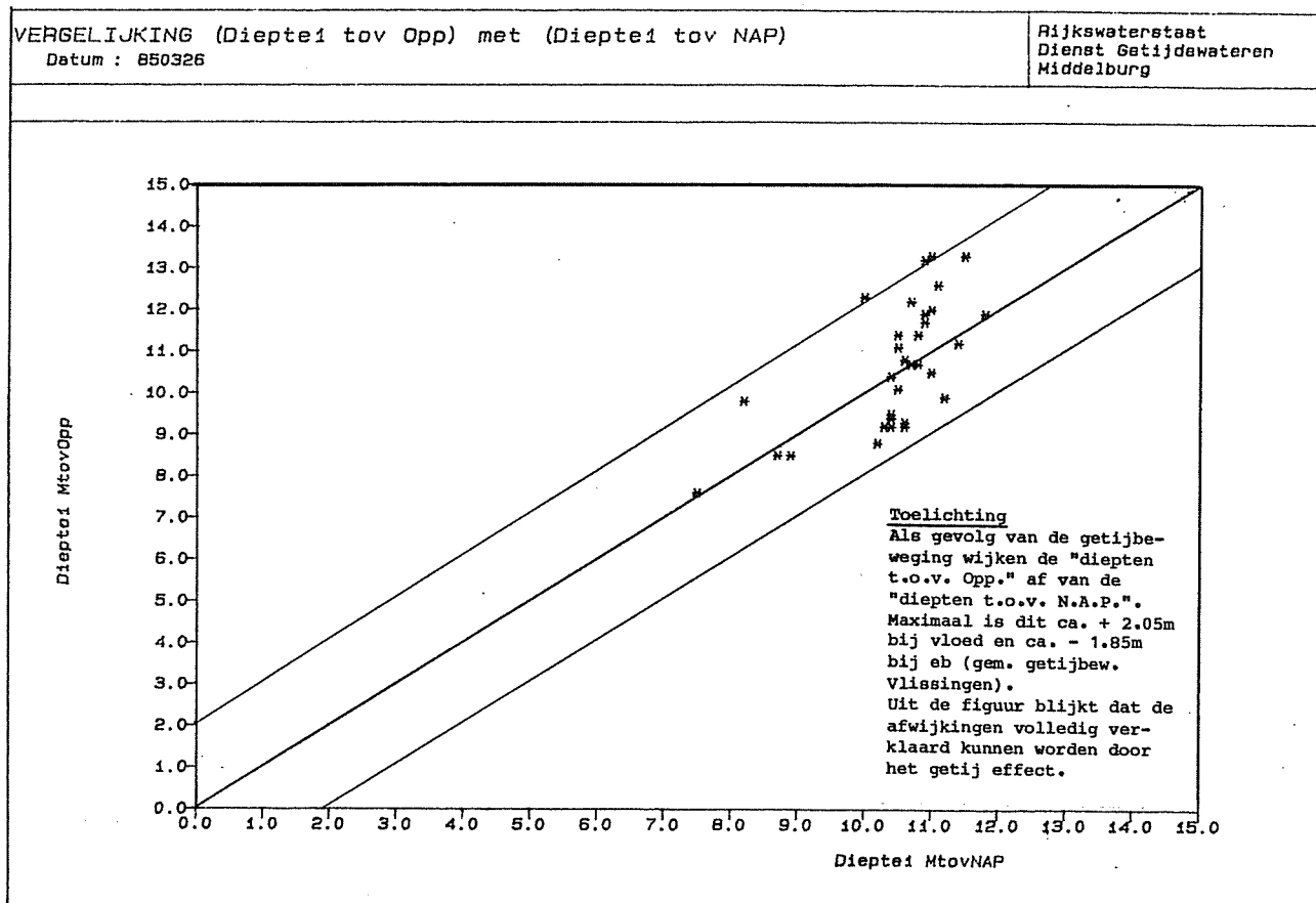
Figuur 4 - Vergelijking "diepte t.o.v. getijwater-oppervlak" met "diepte t.o.v. NAP" voor 56 (25 + 31) stations.
