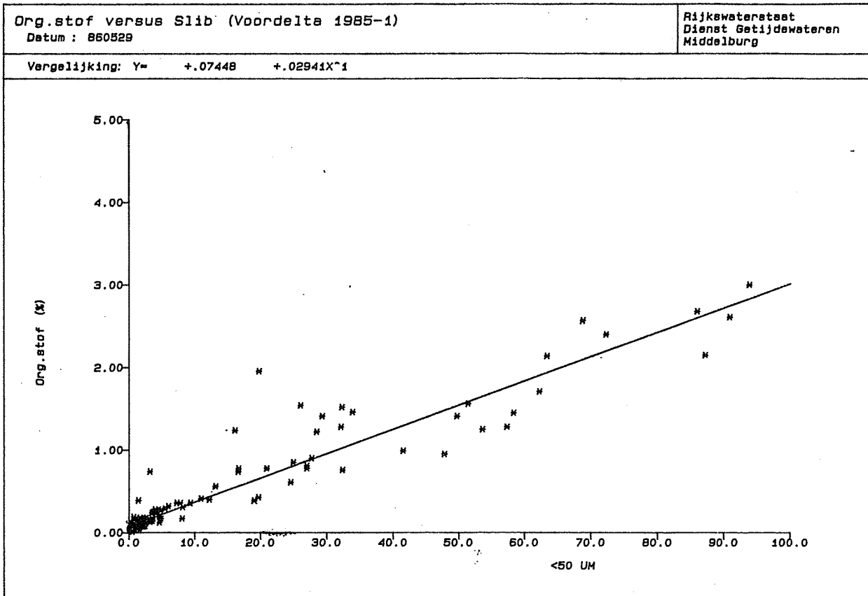
Figuur 3 - Organische stof gehalte (% D.S.) versus slib <50 µm (t.o.v. minerale delen) a.d.h.v. ca 200 Voordelta 1985-1 bodemonmonster data.
