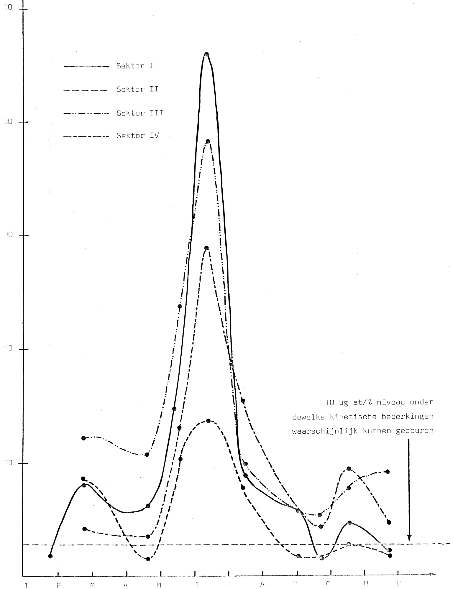
( \mu\text{g N}/\ell ) Fig. I : Seizoenvariatie van nitraat en nitriet ( \mu\text{g}/\ell )
