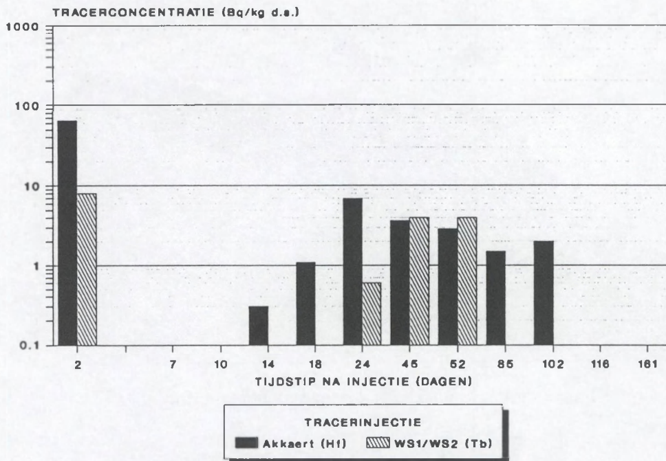
Figuur 3 : Tijdsevolutiegrafiek in de haven van Zeebrugge.
