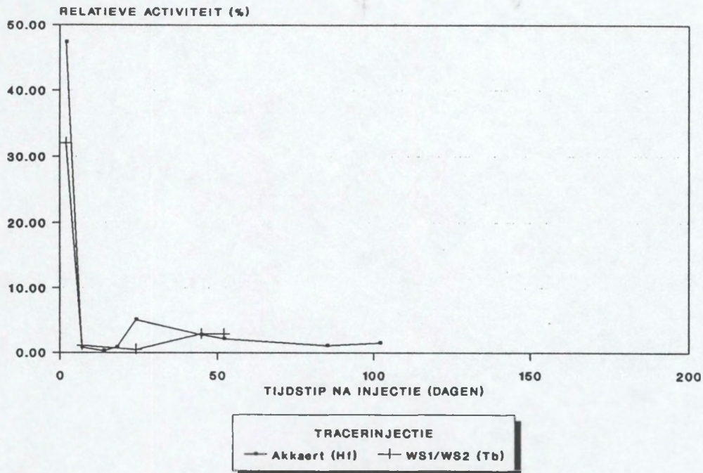
Figuur 5 : Activiteitsdiagram in de haven van Zeebrugge.
