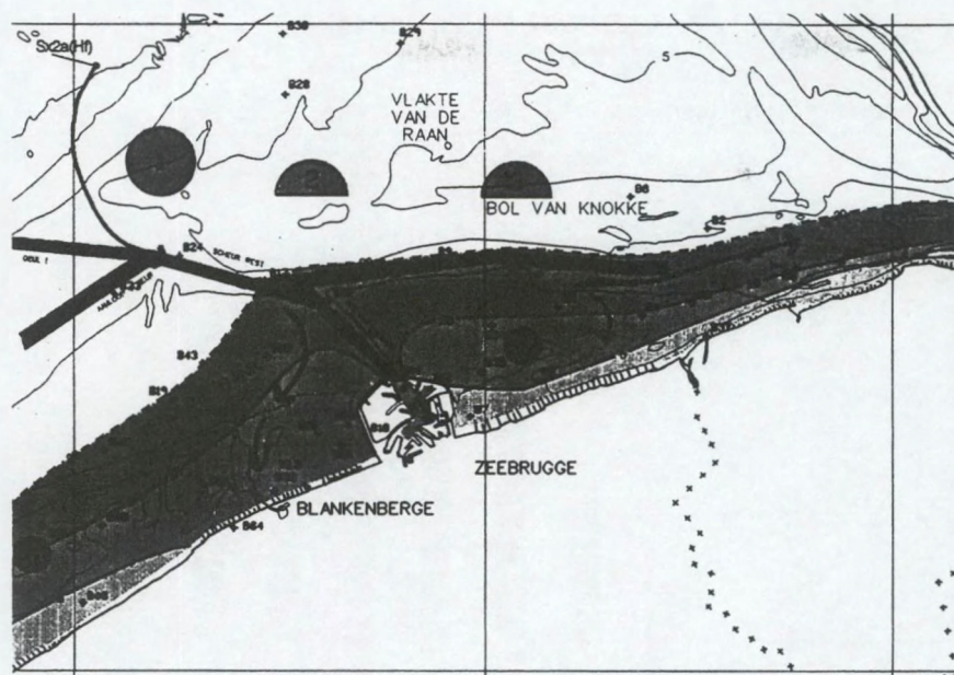
Figuur 4 : Tracerverspreidingskaart, 4 dagen na injectie t.h.v. S1/S2.
