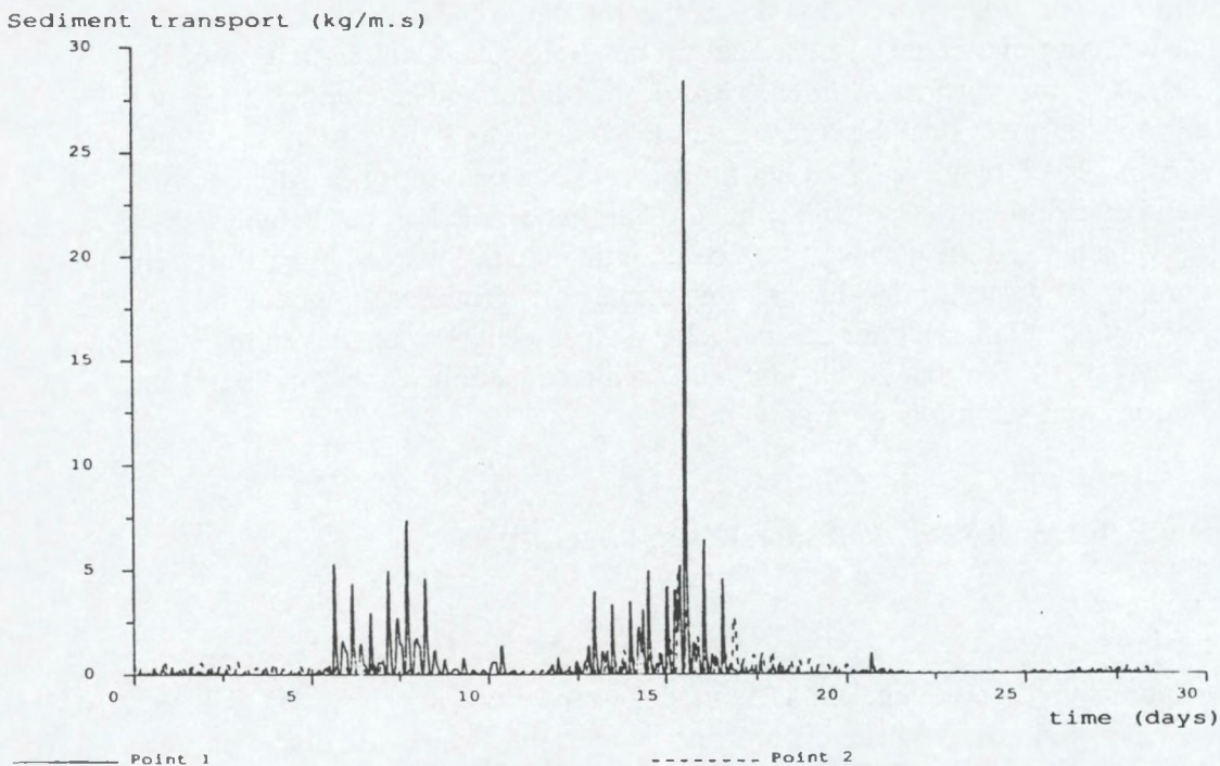
Figuur 4: Ogenblikkelijk sedimenttransport in twee punten
