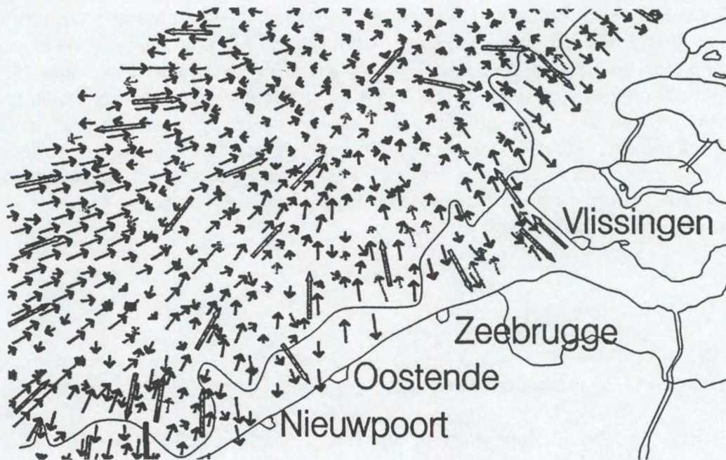
Figuur 6 : Residueel sedimenttransport berekend met STA.
