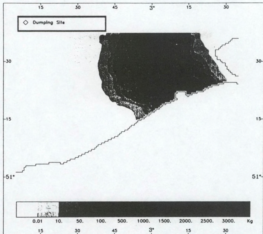
Figuur 13: Resultaten van het model mu-BCZS : een eenvoudig Euleriaans sedimenttransportmodel: massa in suspensie, wanneer alleen advection in rekening wordt gebracht.
