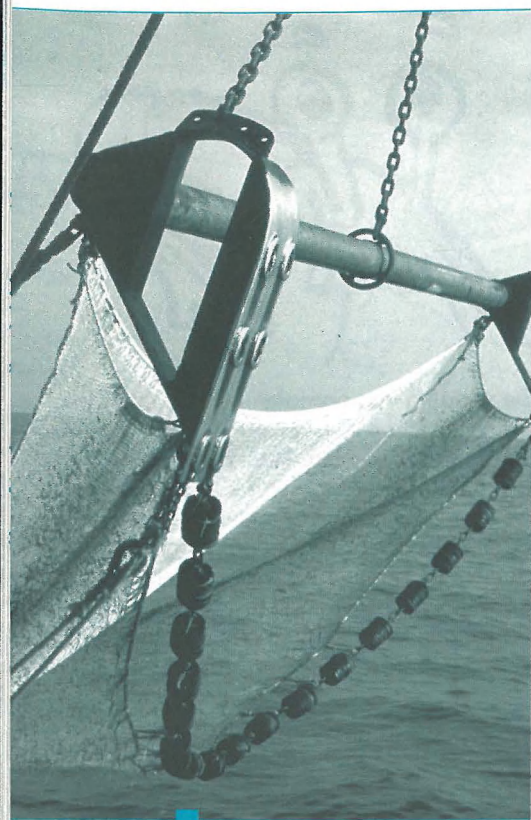
Boomkor met garnaalnet, zoals gebruikt in de beroepsvisserij
