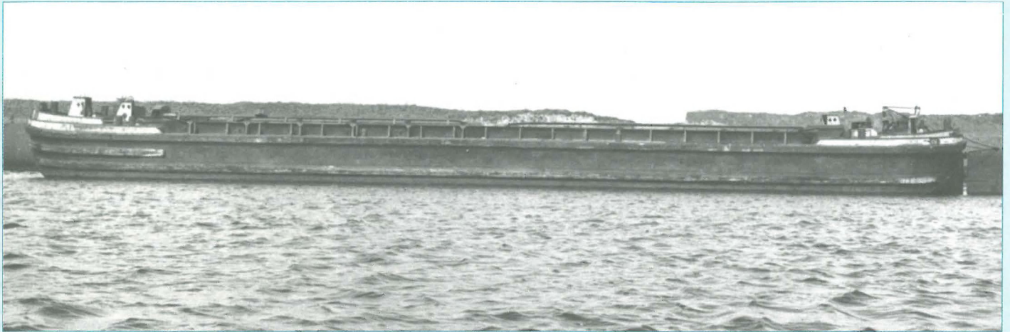
Zogenaamd 'klepbakship', gebruikt voor de dumpingsoperatie van oude WOI munitie vóór de Belgische kust. Zo werd gedurende een half jaar, van november 1919 tot mei 1920, dagelijks een scheepslanding munitie (zo'n 340 ton) in zee gedumpt
