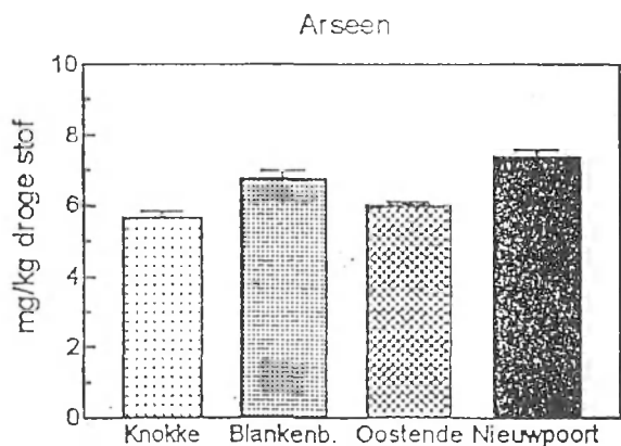
Fig. 7. Concentraties aan zware metalen in mossel 1995-1997 (gemiddelden en standaardafwijkingen in mg/kg droge stof)
