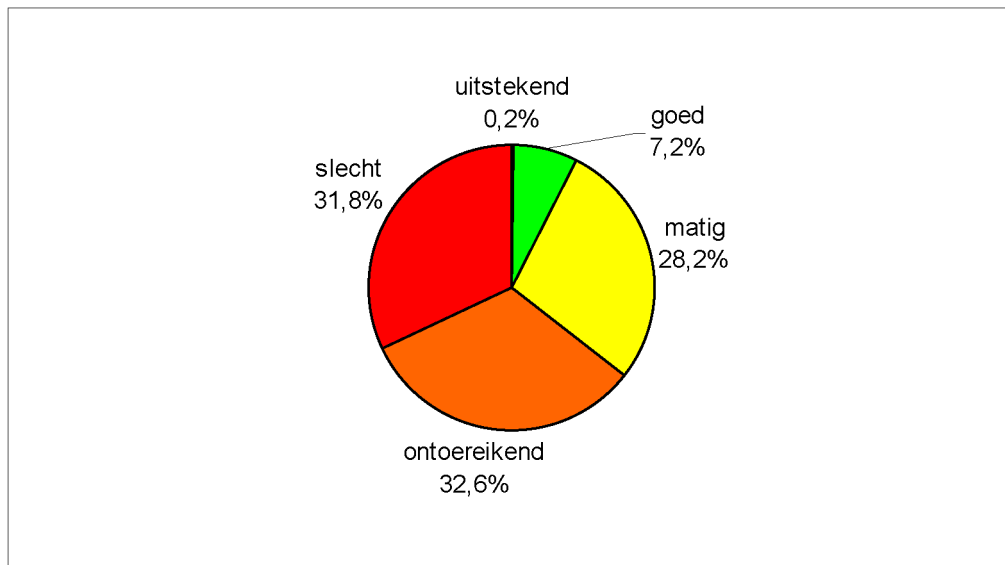
Figuur 26: Biotische integriteit (berekend op basis van EKC) van 663 vismeetpunten (Vlaanderen, 2004-2009)
