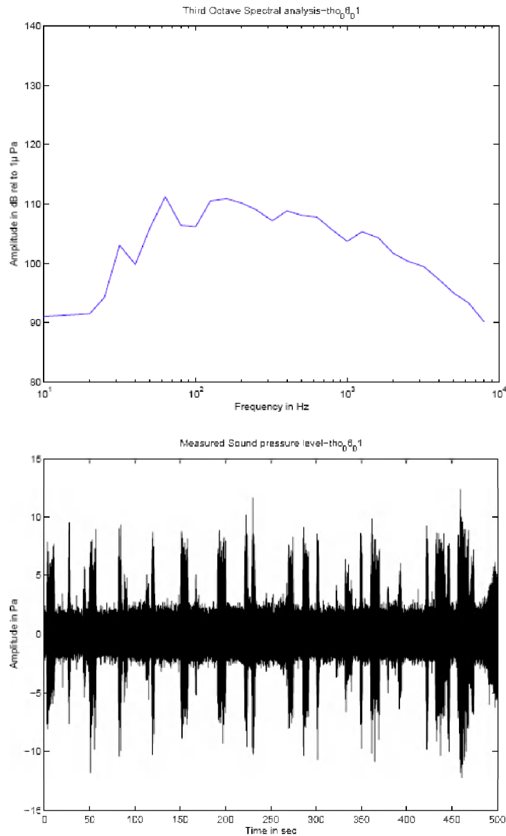
Figuur 5.13: Frequentiespectrum en geluidsdrukniveau op de Thorntonbank op 10 september 2008.
