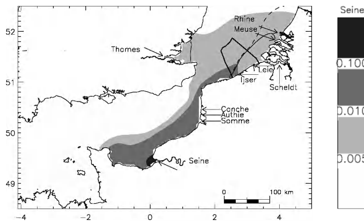
Figuur 2.7: Relatieve distributie van de watermassa's afkomstig van de Seine en andere Franse rivieren (gemiddeld) over de periode 1993-2003 (grijsschaal: 0,5 %, 1 %, 10 %) volgens het model van Lacroix et al. (2004).
