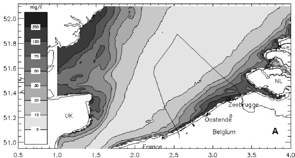
Figuur 2.8: Diepte gecorrigeerde concentratie aan suspensiemateriaal (mg/l) in de zuidelijke Noordzee, afgeleid van 370 SeaWiFS beelden (1997-2002) en in situ metingen, (Fettweis et al. 2007).
