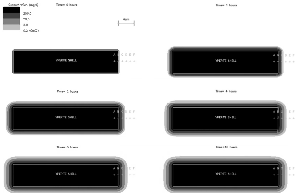
Figuur 5.11: Concentratie van opgelost Yperiet in en rondom de obus (horizontaal vlak) na 0, 1, 2, 4, 8 en 16 uur.
