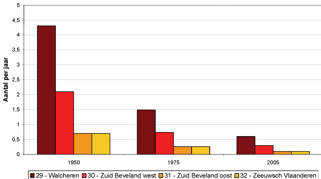
Figuur 8: Geschatte slachtofferrisico's (aantal per jaar) voor de dijkkringgebieden langs de Westerschelde 1950, 1975 en 2005. Bron: van der Klis et al. , 2005 [14]
