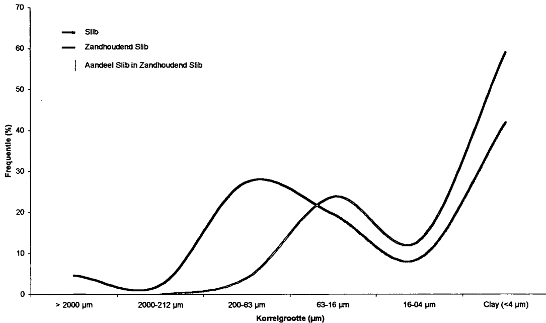
Figuur 5: Bepaling van het aandeel slib (geel oppervlak) in zandhoudend slib (blauwe lijn) door vergelijking met de frequentie-distributie van een kalibratiemonster slib (rode lijn).
