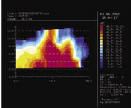
Verticale doorsnede van een stormkern. De afstand op de grond en in de hoogte zijn uitgedrukt in kilometer. De storm strekt zich verticaal tot meer dan 10 kilometer hoogte uit. (© KMI)
