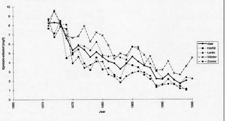
Fig. 15: Seizoens- en jaargemiddelden van Kjeldahl-stikstofconcentraties te Doel boei 87 (Belgisch-Nederlandse grens).
