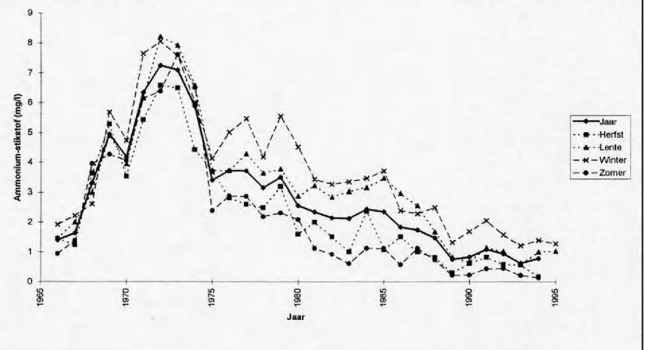
Fig. 14: Seizoens- en jaargemiddelden van ammoniumconcentraties te Doel boei 87 (Belgisch-Nederlandse grens).
