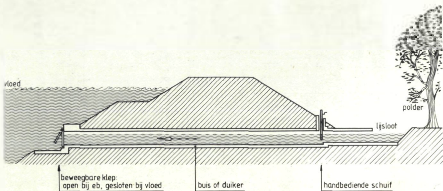
Schema uitwateringssluis
