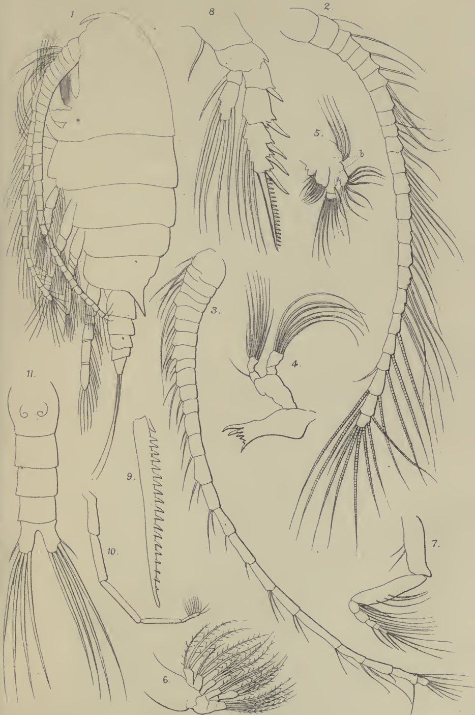
Pseudocalanus armatus.
