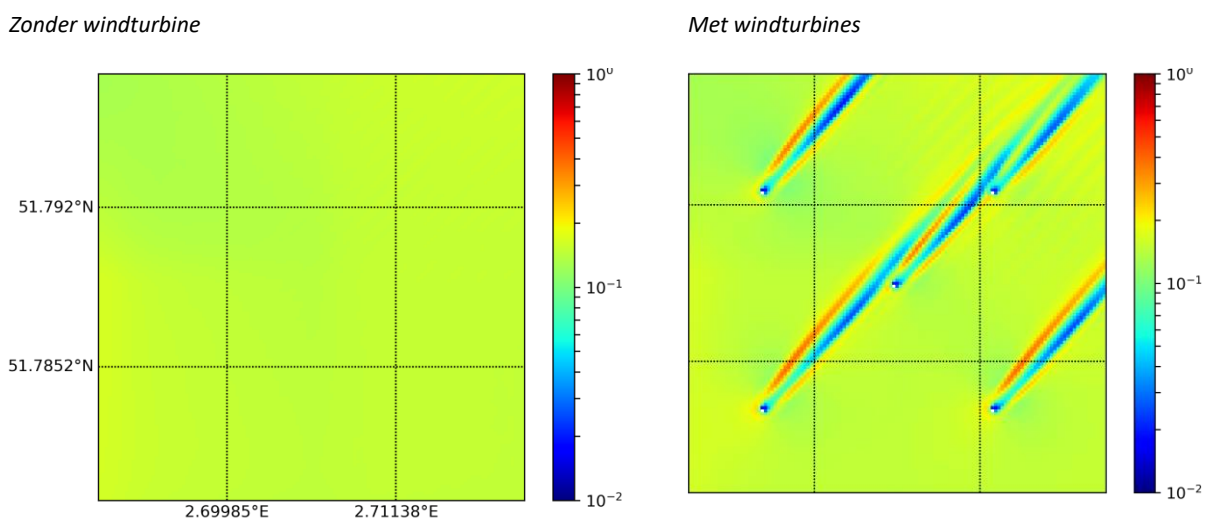
Figuur 2.28. Turbulente kinematische viscositeit ( \text{m}^2/\text{s} ) op \frac{1}{4} hoogte van de waterkolom (op +/- 26,5 m van de bodem) tijdens vloed.
