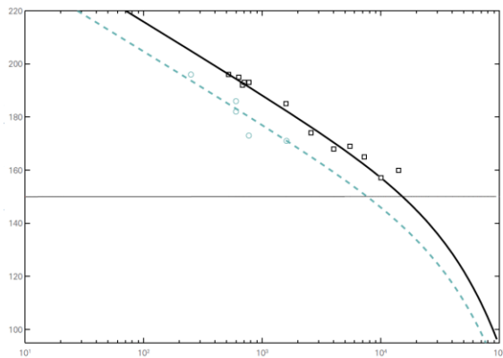
Figuur 2.70. L_{z-p} (dB re 1\mu\text{Pa} ) tegenover afstand van de bron (m, X-as) zoals gemodelleerd voor monopiles (lijn) en jacket funderingen (stippellijn); de metingen zelf zijn aangegeven met vierkantjes (monopiles) en cirkels (jacketfunderingen); het verwachte niveau en bijhorende afstand voor een belangrijke verstoring van bruinvissen volgens Bailey et al (2010) wordt aangegeven door een horizontale lijn (Norro et al., 2013b).
