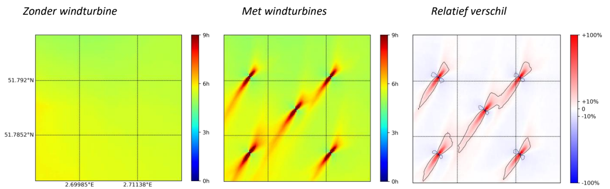
Figuur 2.27. Gemiddelde tijd per getijdencyclus die bevorderlijk is voor de sedimentatie van zand met gemiddelde korrelgrootte ( d \approx 300\mu\text{m} ).
