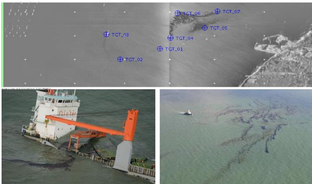
Figuur 2.41. SAR-beeld van eerste grote olieverontreiniging op 06/10/15, aangevuld met een foto van de Flinterstar en van de grote olievlek waargenomen diezelfde dag.
