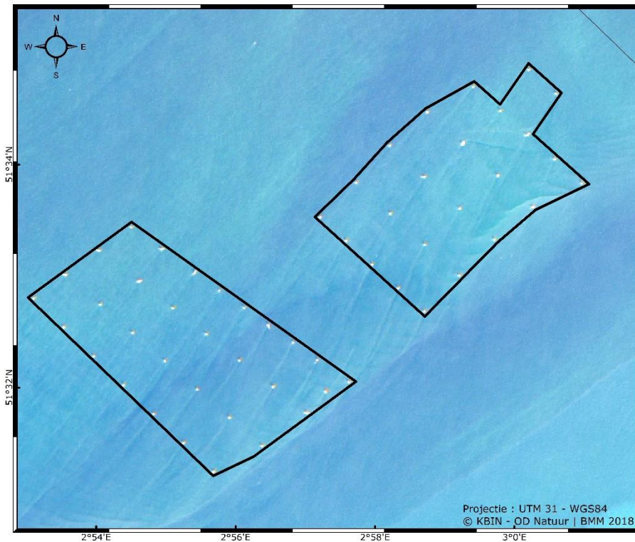
Figuur 2.23. Turbiditeitspluimen die zich ontwikkelen in het zog van de windturbines van het C-POWER park, waargenomen door satelliet Landsat-8 op 7 juni 2015 ("pan-sharpened L8 images", resolutie 15 m per pixel).
