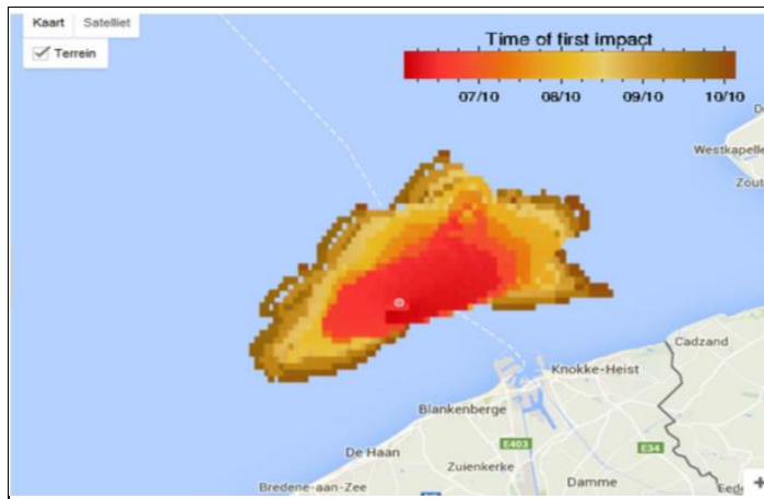
Figuur 2.45. OSERIT 60u-simulatie van spreiding van de 'Flinterstar' olieverontreiniging op de zeebodem.
