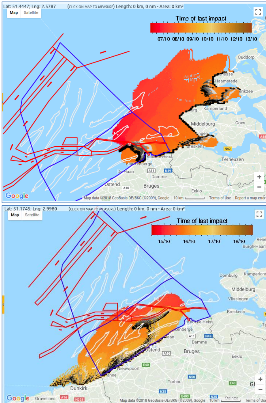
Figuur 2.43. Boven: OSERIT modelsimulatie 08/10/2015, en onder: OSERIT modelsimulatie 15/10/2015, die het mogelijk afrijven van nieuwe olieplekken afkomstig van de Flinterstar aantoont in die periodes.
