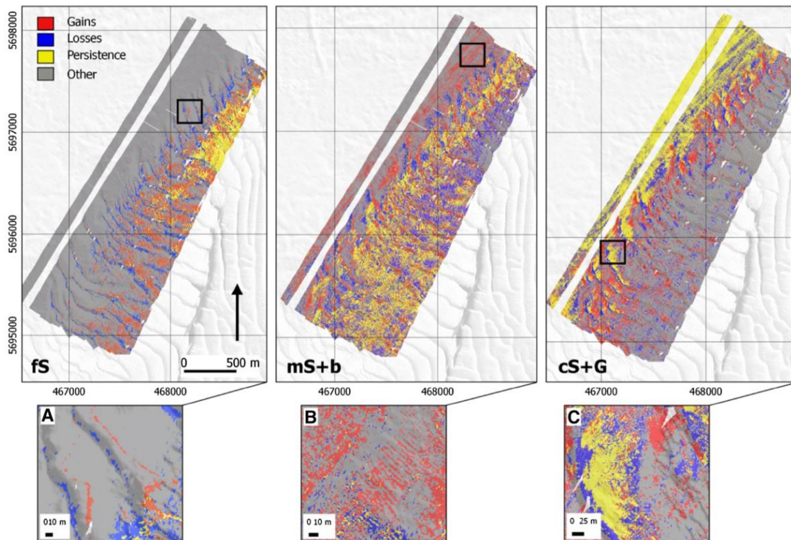
Figuur 2.22. Veranderingen (2010 versus 2014) in het ruimtelijk voorkomen van zeebodemklassen in enkele grindbedden in de Hinder Banken (fs: fijn zand; mS+b: middelgrof zand met schelpenmateriaal; cS+G: grof zand en grind) in termen van winst, verlies en behoud in ruimtelijk voorkomen (Montereale-Gavazzi et al., 2017).
