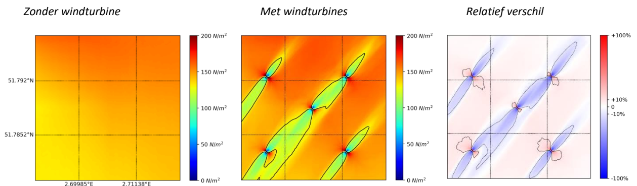
Figuur 2.29. 90-percentiel van de kinetische energie als gevolg van stromingen bij de zeebodem. In het zog van de windturbines kan een afname van de beschikbare kinetische energie op de bodem optreden, die voldoende is om deze zones te laten omschakelen van een "matig energetisch" naar een "laag energetisch" stelsel. De grens tussen beide energiestelsels wordt aangegeven door de zwarte lijn.
