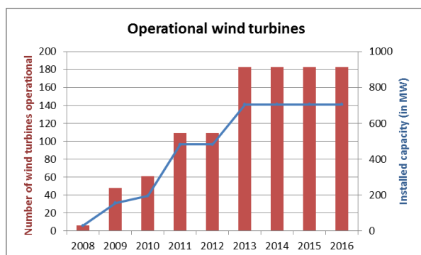
Figuur 2.77. Aantal windturbines (cumulatief) en hun totaal geïnstalleerde vermogen (cumulatief) tussen 2008 en 2016
