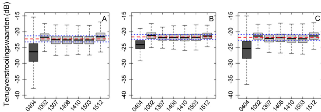
Figuur 2.20. Variatie in de terugverstrooiingswaarden (dB) (gemiddeld per deelgebied, Figuur 2.13) in de periode 2004 tot 2015 (x-axis: jjmm), in enkele grindbedden in de Hinder Banken (RV Belgica EM3002D). Rode en blauwe gestipte lijnen geven respectievelijk een gewogen gemiddelde en \pm 1 \sigma fout op de metingen. Het grote verschil in waarden tussen 0404 en de andere tijdsmomenten is het verschil in multibeamechosounder (Montereale-Gavazzi et al., 2017).
