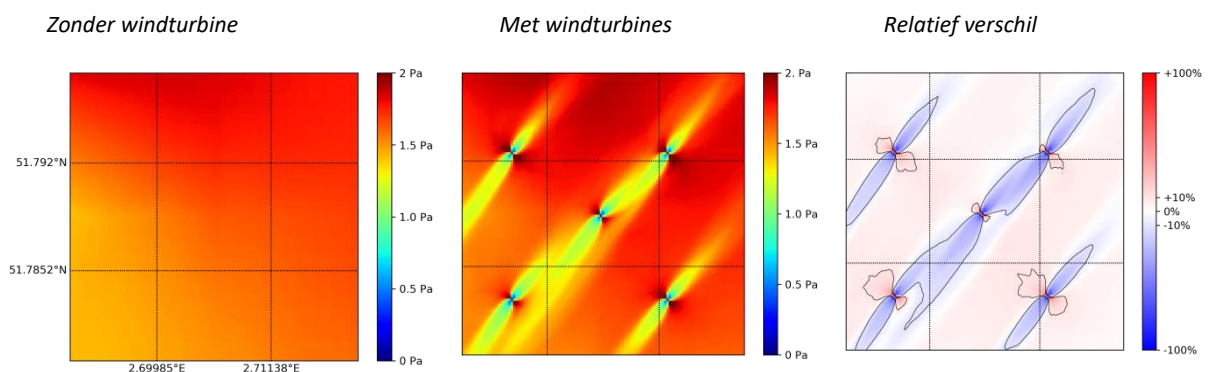
Figuur 2.25. 90-percentiel van de schuifspanning op de bodem.
