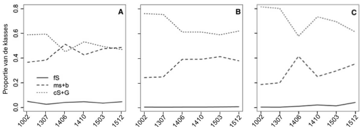
Figuur 2.21. Kartering van de onderlinge verhouding van de sedimentklassen fijn zand (fs), middelgrof zand met schelpenmateriaal (ms+b), en grof zand en grind (cS+G) in de periode 2010 tot 2015 (x-axis: jjmm), in enkele grindbedden in de Hinder Banken (per deelgebied, zie Figuur 2.13) (RV Belgica EM3002D). Merk op dat de toename/afname van grof zand en grind vooral gepaard gaat met een verandering in het voorkomen van gemiddeld zand met bioklastisch materiaal (Montereale-Gavazzi et al., 2017).
