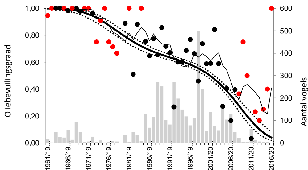
Figuur 2.34. Veranderingen in de oliebevuilingsgraad (linker Y-as) van zeekoeten gevonden langs de Belgische kust in de periode 1961–2017. De bollen tonen de oliebevuilingsgraad en de dunne grillige lijn toont het verloop van het vijfjarig gemiddelde. Wanneer er minder dan 25 individuen werden gevonden, werd een bol rood gekleurd, anders zwart. De grijze balken tonen het aantal individuen waarop de oliebevuilingsgraad is gebaseerd (rechter Y-as). De dikke zwarte lijn en de bijbehorende gestippelde betrouwbaarheidsintervallen zijn het resultaat van een GLM-regressie.
