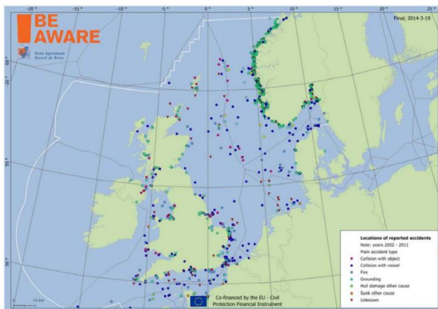
Figuur 2.48. Geografische spreiding van de 1069 ongevallen op zee zoals gerapporteerd in de zone van de akkoorden van Bonn tussen 2002 en 2011
