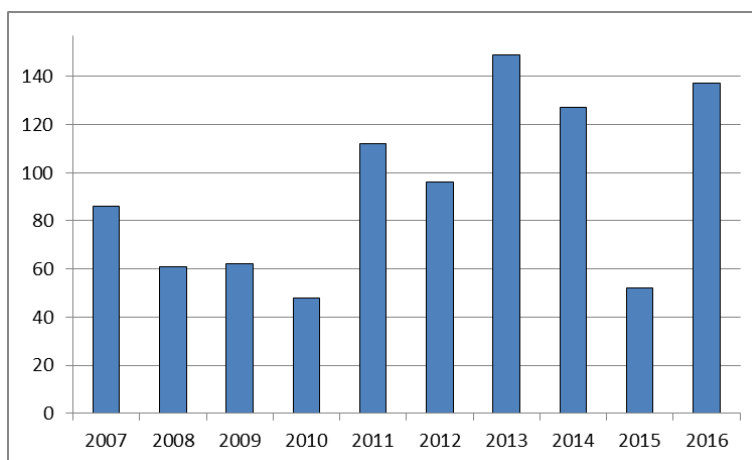
Figuur 3.10. Jaarlijks aantal angespoelde bruinvissen (2007-2016) (data KBIN)
