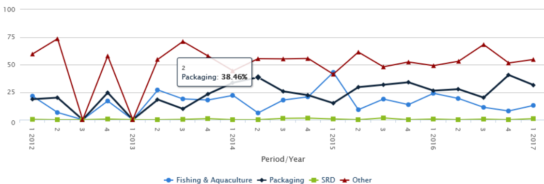
Figuur 2.59. Afvalbron (%) per seizoen per jaar voor de Belgische stranden (Oostende Halve Maan, Raversijde) tussen 2012 en 2017 (Bron: OSPAR)
