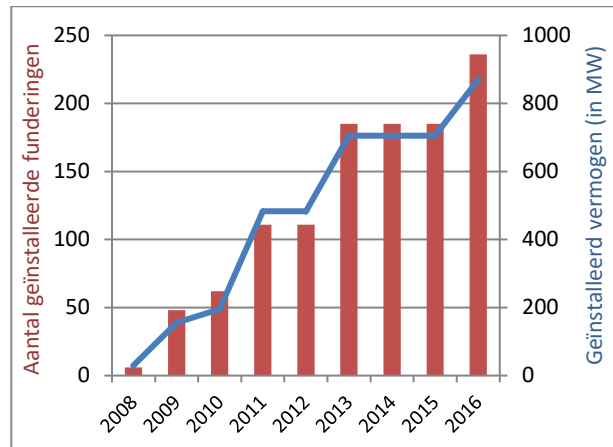
Figuur 2.72. Aantal geïnstalleerde funderingen (cumulatief) en geïnstalleerd vermogen (cumulatief) tussen 2008 en 2016
