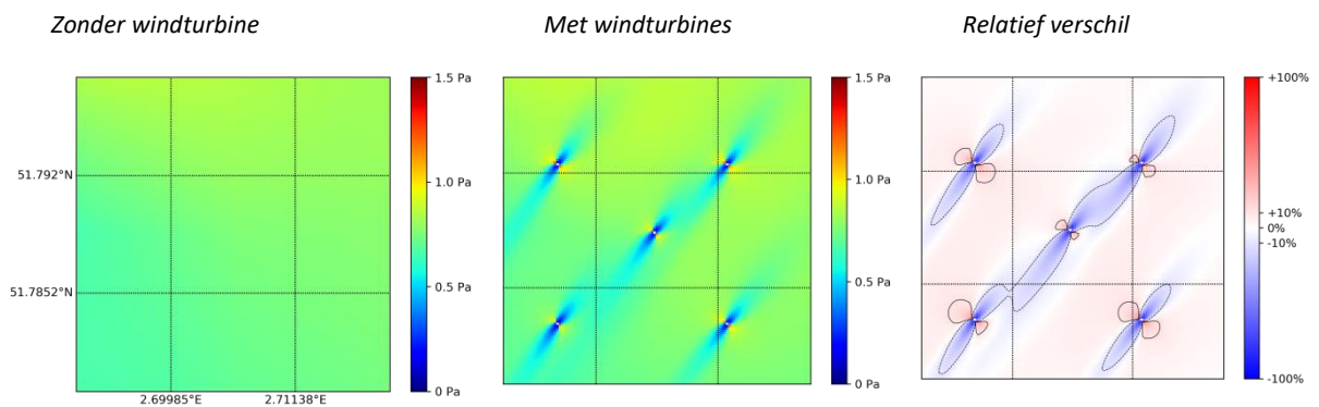
Figuur 2.24. Gemiddelde schuifspanning op de bodem over een getijdencyclus. De aanwezigheid van windturbines veroorzaakt een weerstand in het zog van de windturbines en een erosiezone aan de voet van elke windturbine. De maximale impact vindt plaats bij de meest intense getijstromingen, zowel bij vloed als bij eb.
