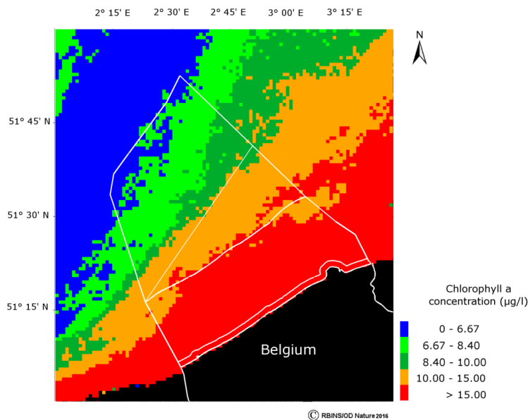
Figuur 2.11. Classificatie van Chl P90 op basis van satellietbeelden (2006-2011) in het BDNZ. De rode zone geeft een Chl P90 > 15 \mu\text{g/l} weer.
