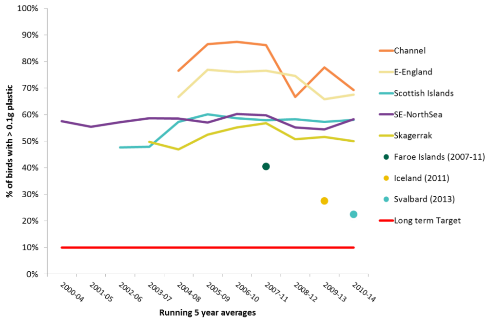
Figuur 2.67. Trend in het percentage vogels (vijfjarig gemiddelde) met meer dan 0,1 g plastic in hun maag, uitgesplitst per regio (overgenomen van OSPAR 2017).
