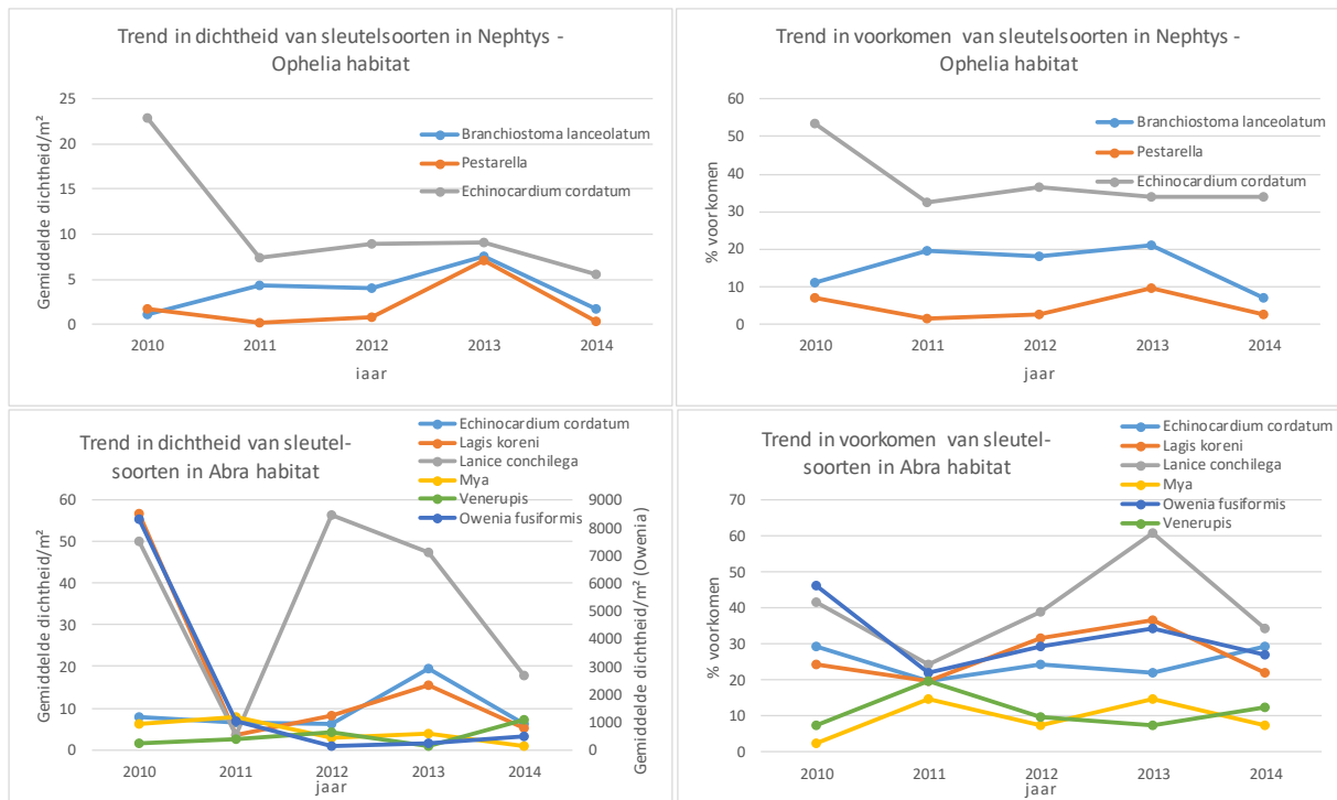
Figuur 3.18. Gemiddelde dichtheid (links) en relatief voorkomen (rechts) van een aantal belangrijke soorten per habitattypen en per jaar.
