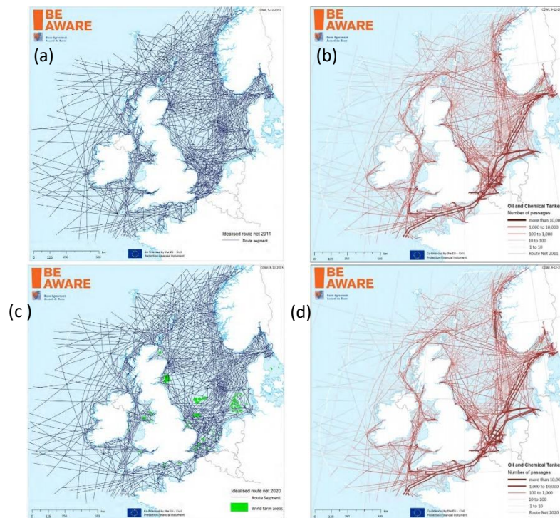
Figuur 2.50. Het netwerk van zeevaartroutes voor het jaar 2011 (a) en de vermoedelijke evolutie ervan in 2020 (c). Dit netwerk deed dienst als drager voor een fijne analyse van het scheepvaartverkeer, bijvoorbeeld door het weergeven van de verwachte evolutie van het verkeer van olie- en chemicaliëntankers tussen 2011 (b) en 2020 (d).
