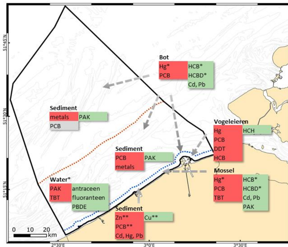
Figuur 2.31. Overzicht van de evaluatie van concentraties aan verontreinigende stoffen voor het BDNZ, kustwateren (1nm), territoriale wateren (tussen 1 en 12nm) en offshore (> 12nm) gebied. Rood: niet goed, overschrijding van de norm; groen: goed. Met * KRW Prioritaire stoffen, **RBS: KRW Scheldespecifieke verontreinigende stoffen.
