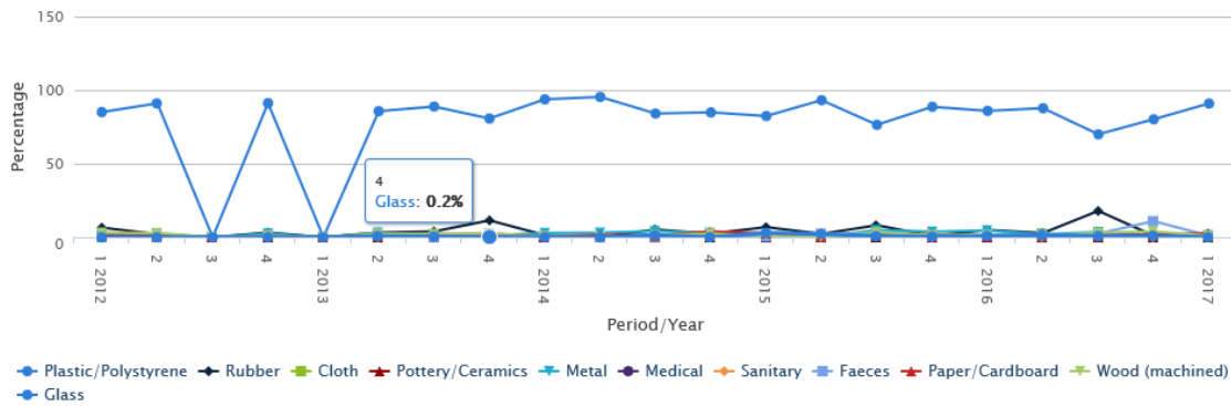
Figuur 2.58. Materiaaltypes (%) per seizoen per jaar voor de Belgische stranden (Oostende Halve Maan, Raversijde) van 01-01-2012 tot 31-01-2017 (Bron: OSPAR)
