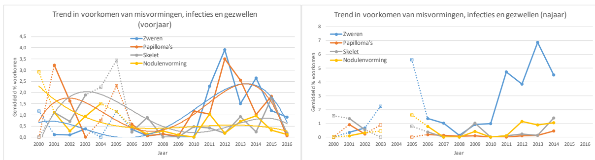
Figuur 2.37. Gemiddeld procentueel voorkomen voor 4 visaandoeningen in schar in voorjaar (links) en najaar (rechts) voor de periode 2000-2016. Voor het voorjaar zijn de polynomiale trendlijnen van de vierde orde weergegeven. Voor najaar niet mogelijk door te veel ontbrekende datapunten. Open punten zijn analyses op minder dan 250 schar individuen.
