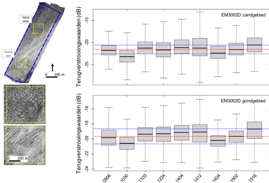
Figuur 2.19. Variatie in de terugverstrooiingswaarden (dB) (gemiddeld over een typisch zand- en grindgebied) in de periode 2009 tot 2015 (x-axis: ijmm), in een grindrijk gebied in de Vlaamse Banken (Figuur 2.13 voor locatie). Rode en blauwe lijnen geven respectievelijk een gewogen gemiddelde en \pm 1\sigma fout op de metingen. Data van RV Belgica EM3002D multibeam echosounder.
