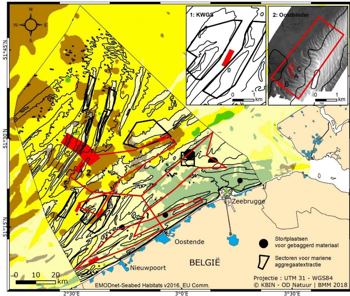
Figuur 2.13. Transecten en deelgebieden die werden gekarteerd met multibeamtechnologie om de evolutie in de distributie van grootschalige sedimenttypes (Figuur 2.12) te kwantificeren. De grindgebieden waar tijdsreeksen van multibeamdata toelieten om de evolutie van hard versus zacht substraat doorheen de tijd te kwantificeren zijn rechtsboven aangeduid
