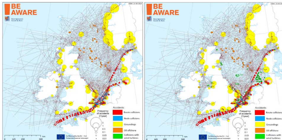
Figuur 2.51. Frequentie van het risico van ongevallen op zee in de Noordzee in 2011 (a) en 2020 (b).
