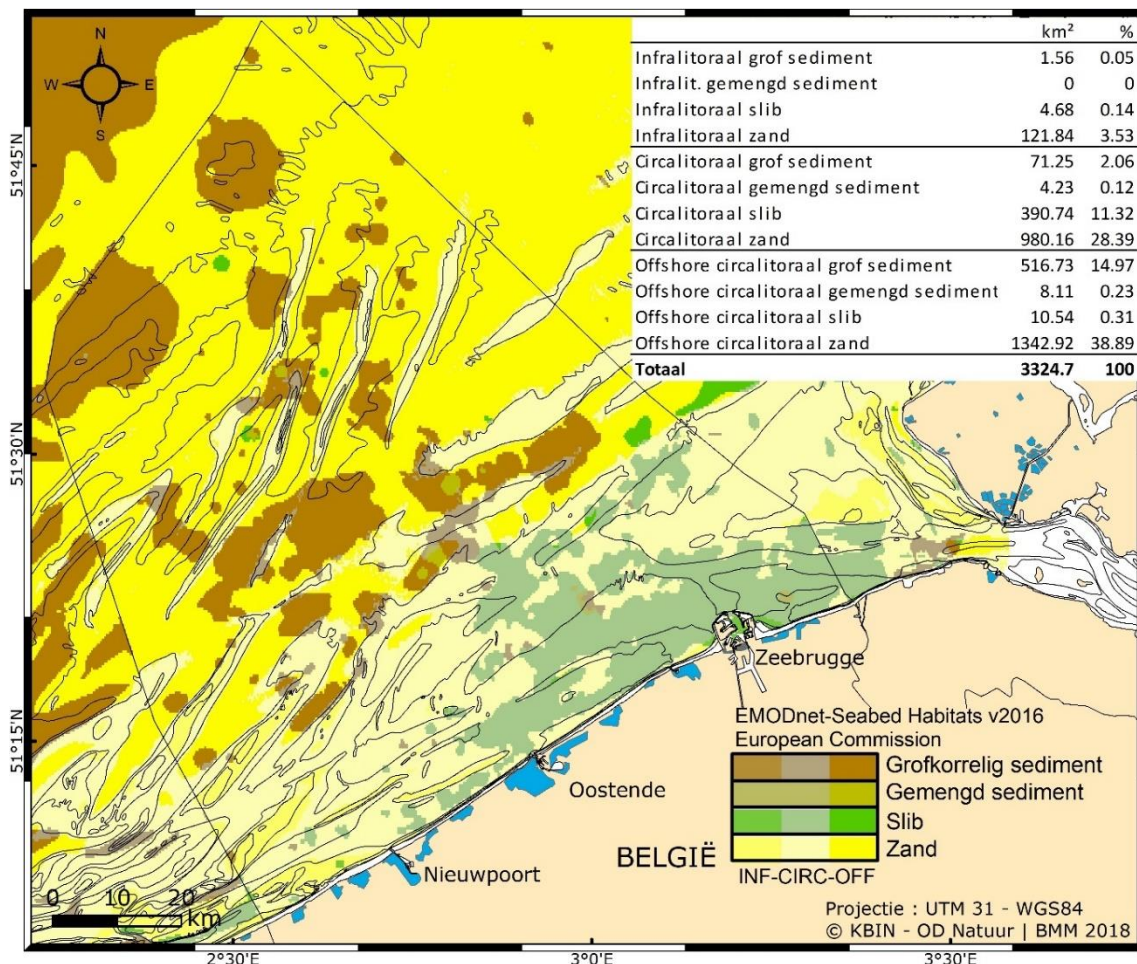
Figuur 2.12. Grootschalige habitattypes waarvan het voorkomen en de distributie in de tijd wordt opgevolgd.
