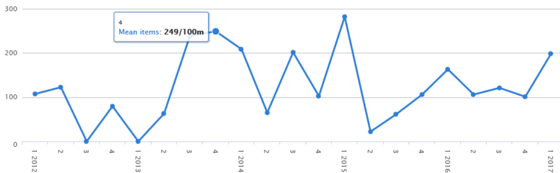
Figuur 2.57. Gemiddeld aantal voorwerpen/100 m per seizoen per jaar voor de Belgische stranden (Oostende Halve Maan, Raversijde) van 01-01-2012 tot 31-01-2017 (Bron: OSPAR)
