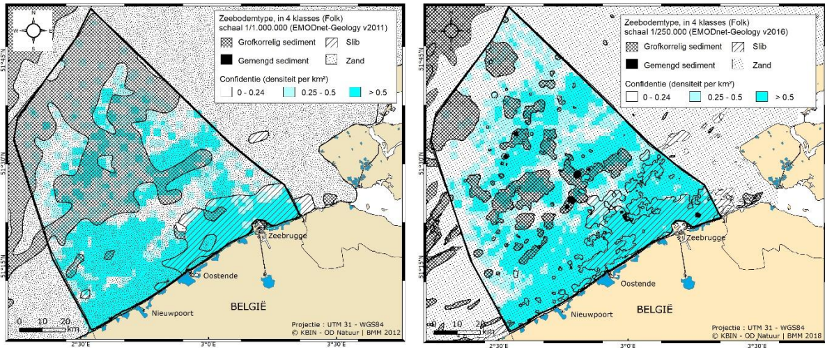
Figuur 2.17. Voorkomen en distributie van de grootschalige sedimenttypes slib, zand en grofkorrelige sedimenten in 2012 (Stevenson et al., 2012) en 2016 (European Commission, 2012b) (Folkclassificatie), alsook een maat van confidentie op basis van puntdensiteit per km 2 .
