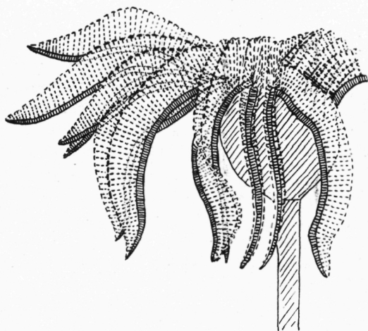
Fig. 1. — Diamenocrinus stellatus JAEKEL. — Schéma basé sur une dissection de la contre-empreinte du spécimen D 1 et illustrant la diversité observée dans la position des bras. \times 6/7 .
