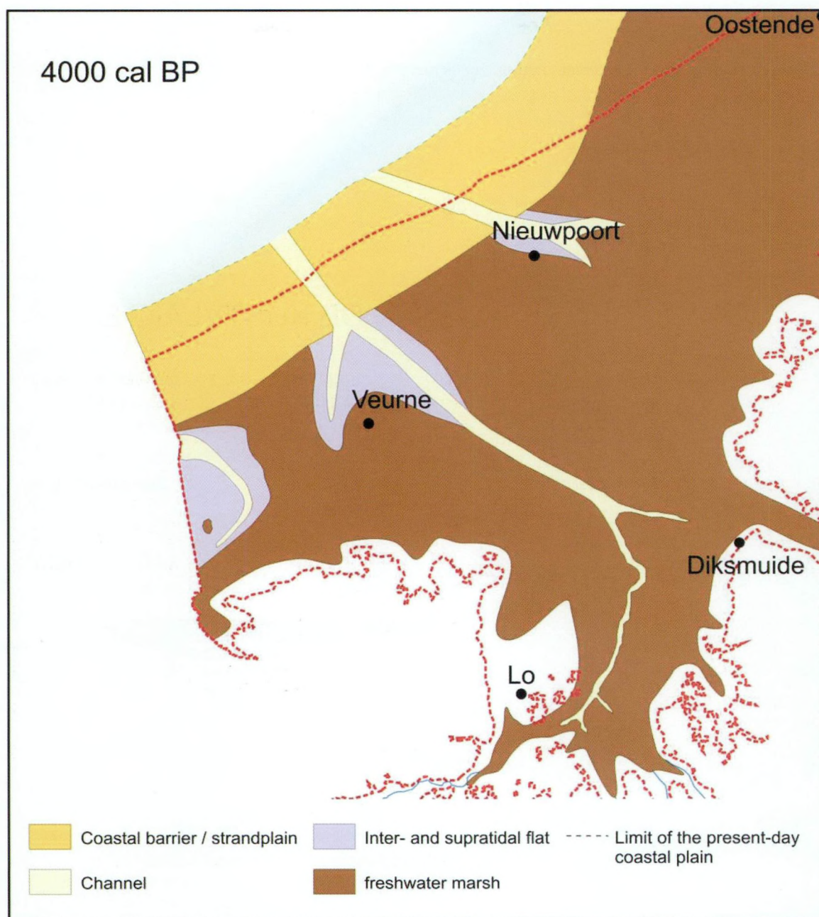
Fig. 6.8 b De paleogeografische reconstructie van de westelijke kustvlakte voor de perioden 6800-6000 cal BP (a) en ca. 4000 cal BP (b) toont het zeewaarts uitbouwen van de kust. Sl: zeeniveau (gemiddeld hoogwater).
