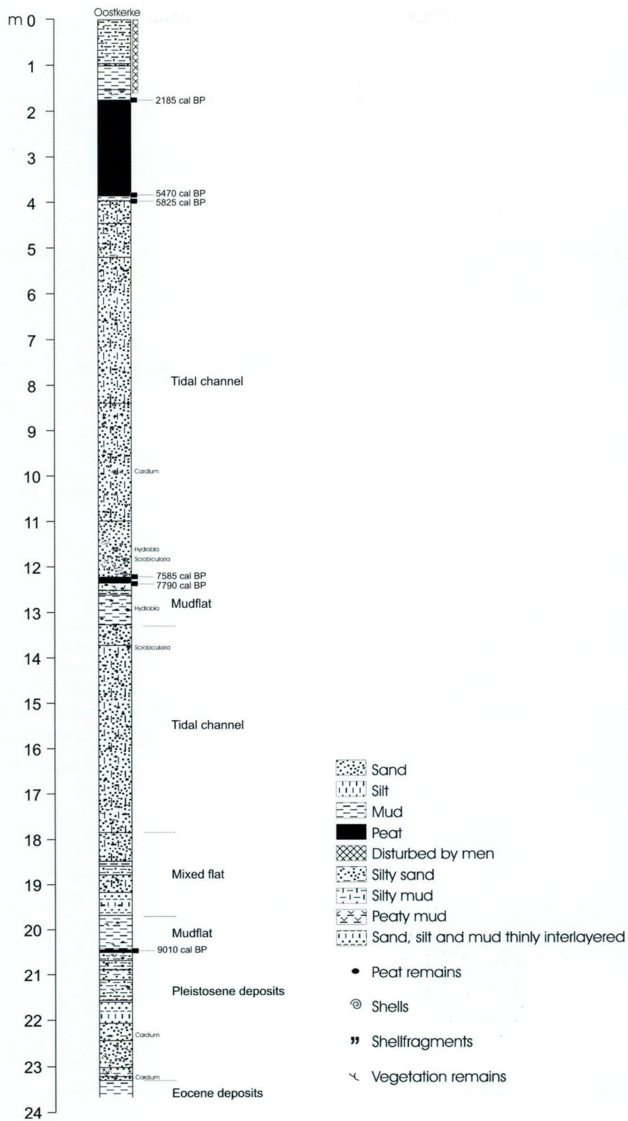
Fig. 5.3 Tekening van de boring Oostkerke.
