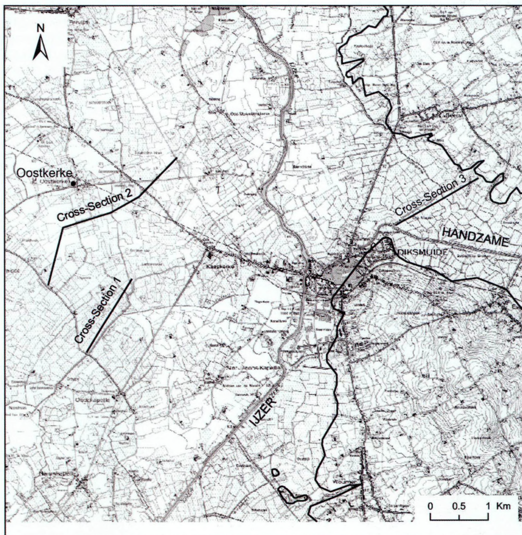
Fig 5.1 Kaart van het centrale deel van de westelijke kustvlakte met locatie van de dwarsdoorsneden en boring Oostkerke.
