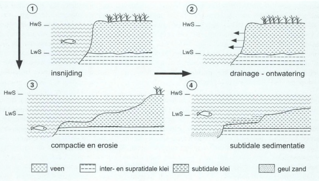
Fig. 3.5 Schematische voorstelling van ontwatering en compactie van het veen door verticale erosie van de laat-Holocene getijdgeulen.
