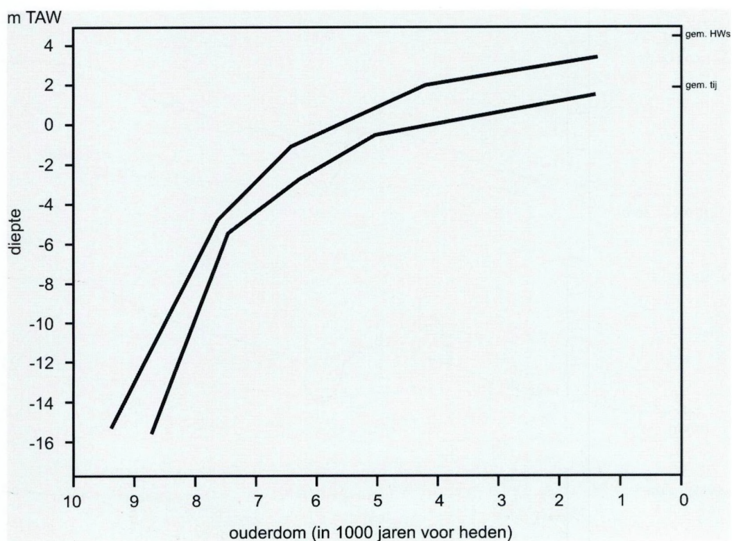
Fig. 3.3 Curve van de relatieve zeespiegelstijging weergegeven aan de hand van een enveloppe voor minimum- en maximumniveau.
