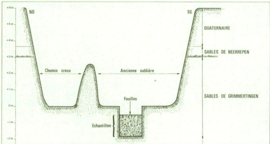
Fig. 1. — Localisation des fouilles faites dans les Sables de Grimmertingen (coordonnées LAMBERT : x = 224.820 ; y = 168.520 ).
