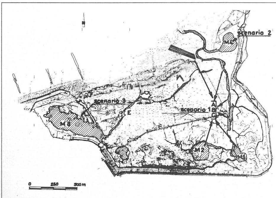
Fig. 6: Het verhogen van de komberging - mogelijke scenario's.
