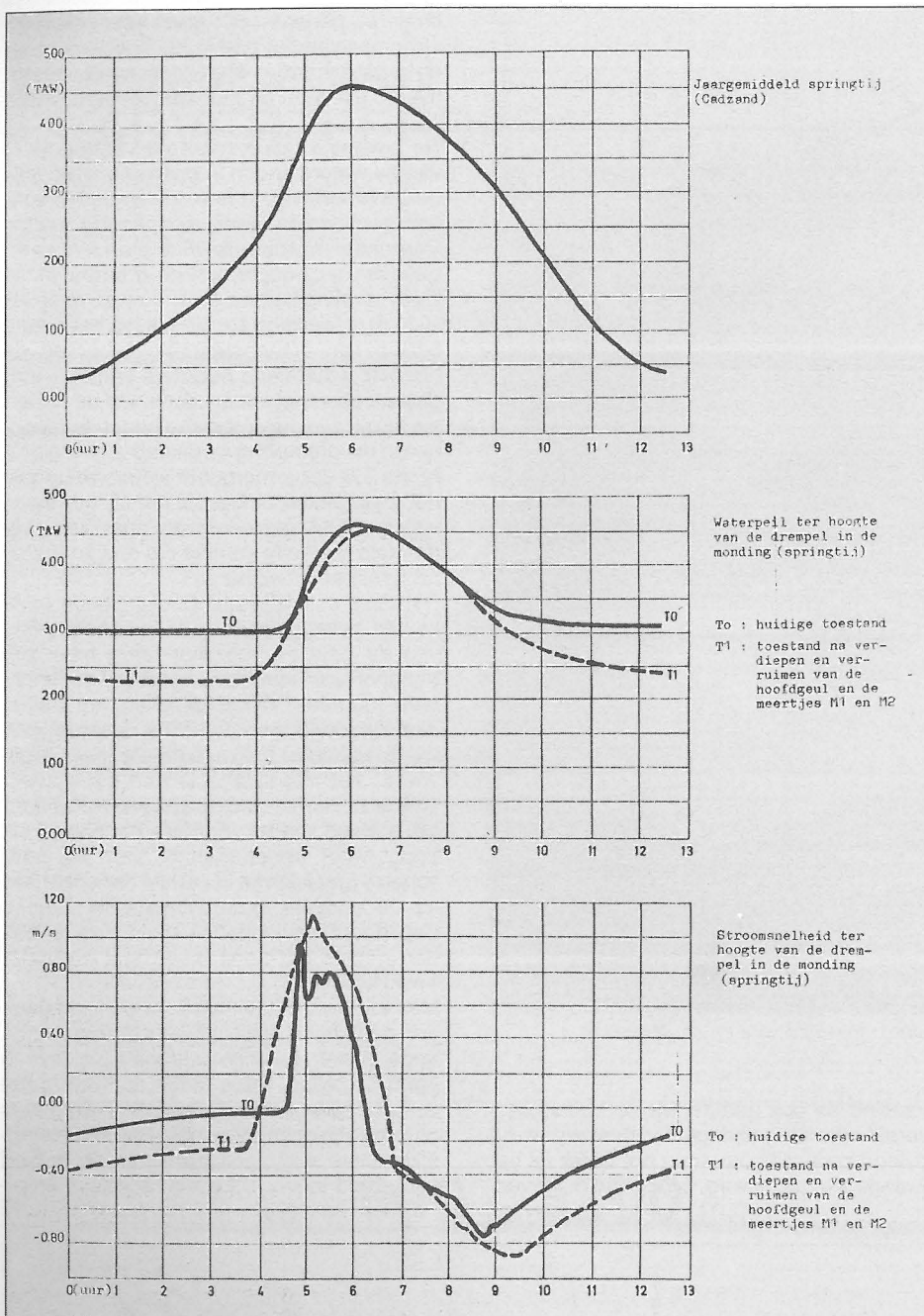
Fig. 3: Relatie tussen de getijdestand in open zee, en de waterstanden en -stroomsnelheden ter hoogte van de geuldrempel in de Zwinmondning.
