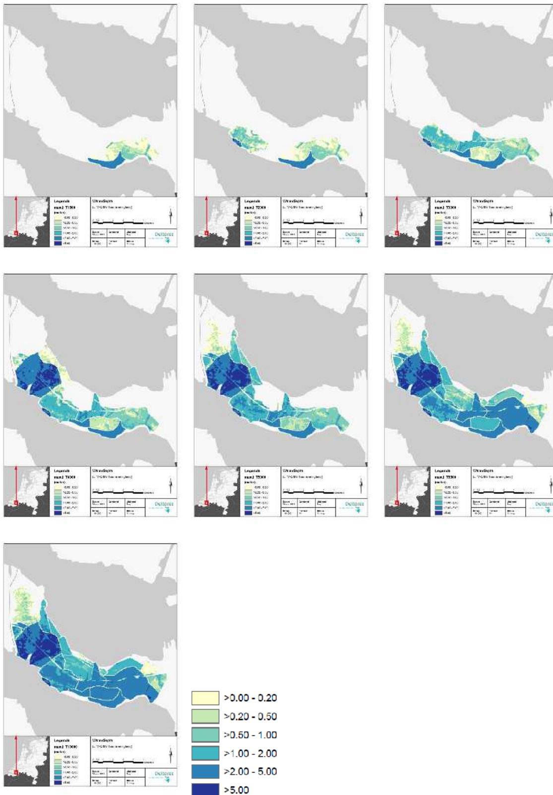
Figuur 4.20 Maximum waterdieptes berekend met SOBEK voor stormvloed en met een kans van voorkomen van 1:1500, 1:2000, 1:3000, 1:4000, 1:5000, 1:6500 en 1:10000 per jaar waarbij de eerder beschreven bressen optreden in een zanddijk.
