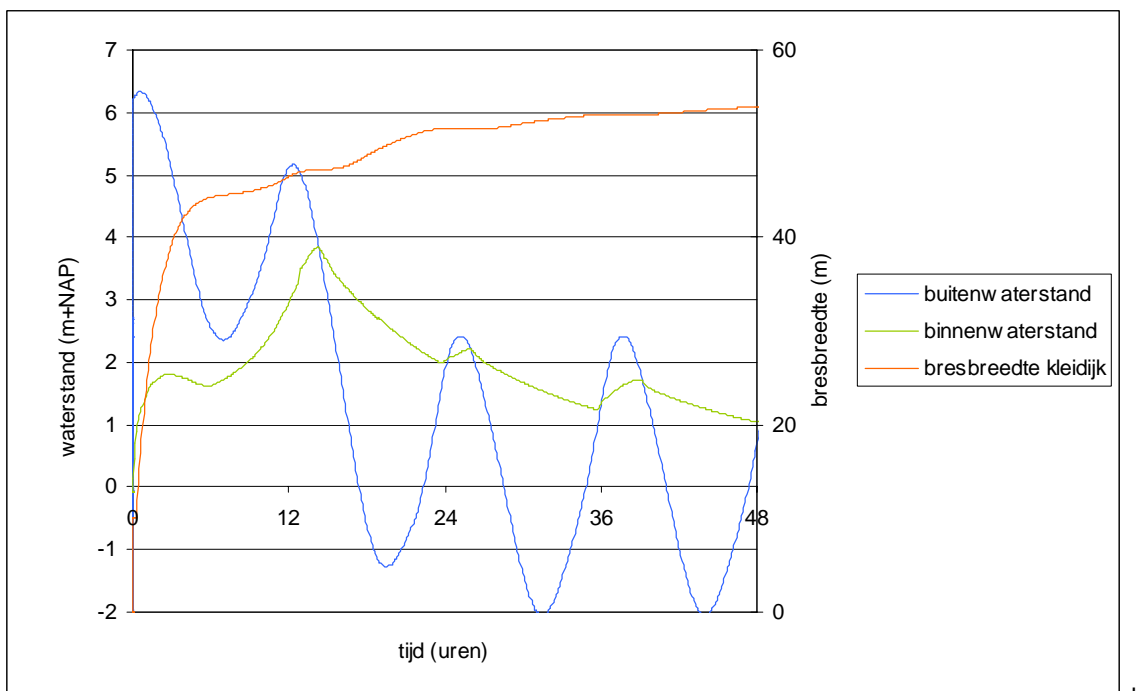
Figuur 4.13 Bresgroei gesimuleerd met SOBEK voor bres 1, tijdens een stormvloed met een kans van voorkomen van 1:10.000 per jaar (a) zanddijk, (b) kleidijk
