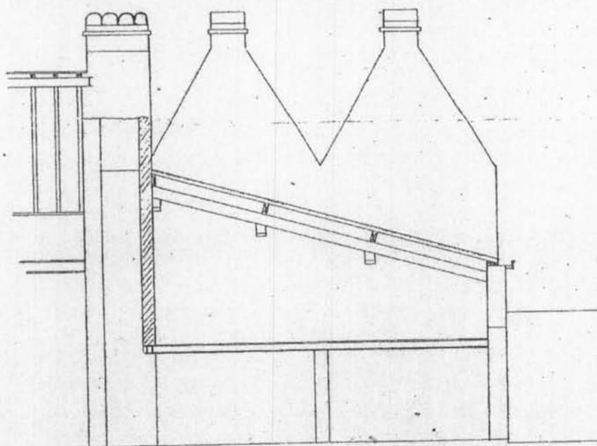
DOORSNEDEN A-B
