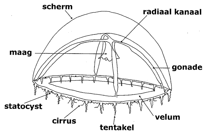
Fig. 1d: Leptomeduse
