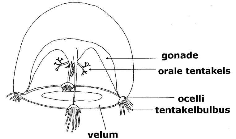
Fig. 1b: Anthomeduse
