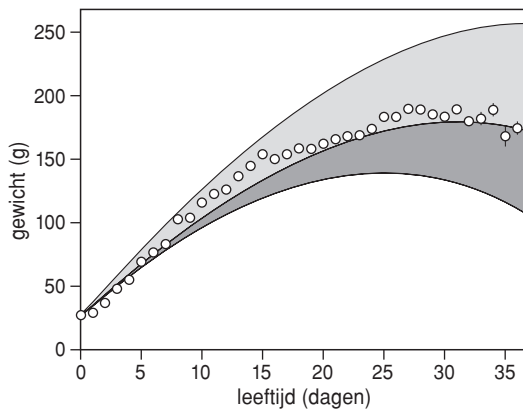
Figuur 1. Mathematisch model van het cumulatieve effect van wind en prooiverlies op de groei van Grote Sternskuikens op Griend. De bovenste getrokken lijn geeft de theoretische groei van een kuiken bij zeer gunstige windomstandigheden (5 m/sec) en wanneer in het geheel geen prooiverlies zou optreden. De middelste lijn toont de groei bij aanhoudende harde wind (15 m/sec) maar eveneens zonder prooiverlies. Wanneer ook nog rekening wordt gehouden met het verlies van prooien o.a. aan rovende Kokmeeuwen (onderste lijn) dan blijft de groei sterk achter bij de werkelijke groei (witte stippen, gemiddelde gewichten \pm SE). Bij aanhoudende harde wind zullen de kuikens het uiteindelijk niet overleven.
