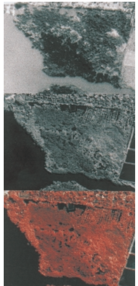
Voor een moeilijk toegankelijk en uitgestrekt biotop als mangrovebossen zijn teledetectie- of 'remote sensing' technieken (luchtfotografie en satelliet-imagery) een ideaal instrument om samenstelling en bedekking op te volgen. Hier een zwart/wit luchtfoto (boven), panchromatisch IKONOS satellietbeeld (midden) en 'pan-sharpened' valse kleurencompositie (onder: blauw/groen/nabij-infrarood) van een weinig veranderde mangroveformatie in Sri Lanka. Te zien is hoe vegetatiestructuurattributen die tot nu toe enkel beschikbaar waren via luchtfotografie nu deels kunnen gedetecteerd worden via satellietbeelden met zeer hoge ruimtelijke resolutie (1 meter)(FDG)
