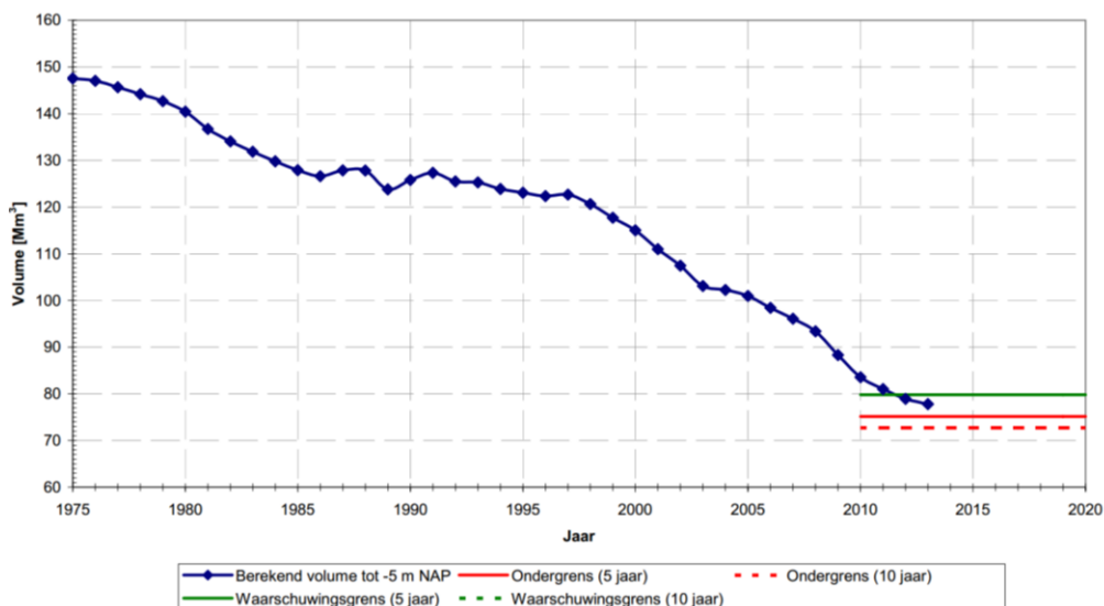
Figuur 2-26: Netto volume nevengeul macrocel 4 (bron: Schrijver, 2014)
