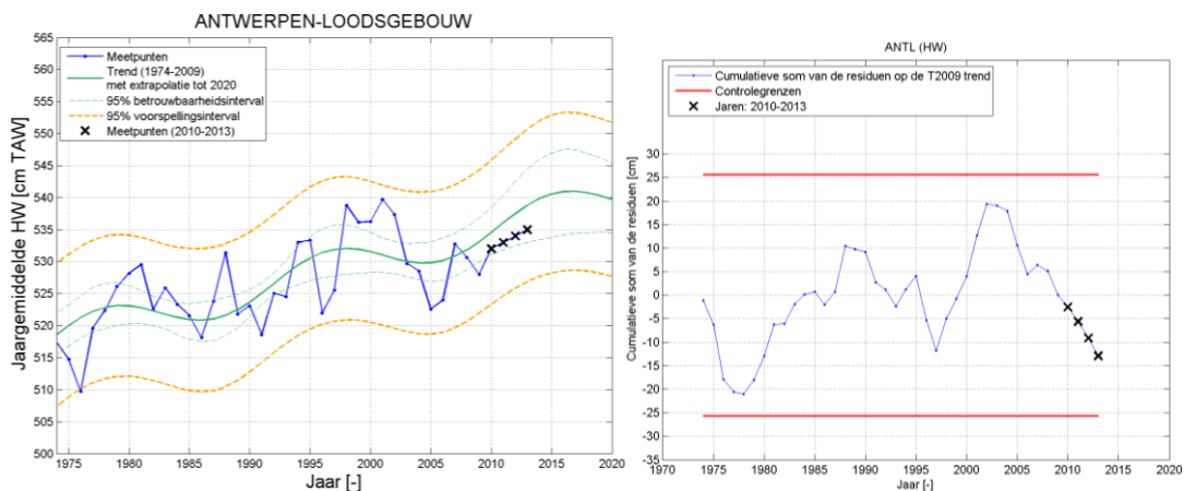
Figuur 2-14: Links: Evolutie van de jaargemiddelde hoogwaterstand te Antwerpen-loodsgebouw, met T2009 trendlijn (extrapolatie tot 2020), 95 % betrouwbaarheids- en verwachtingsinterval. Rechts: Cumulatieve som van de residuen op de (geëxtrapoleerde) T2009 trend.
