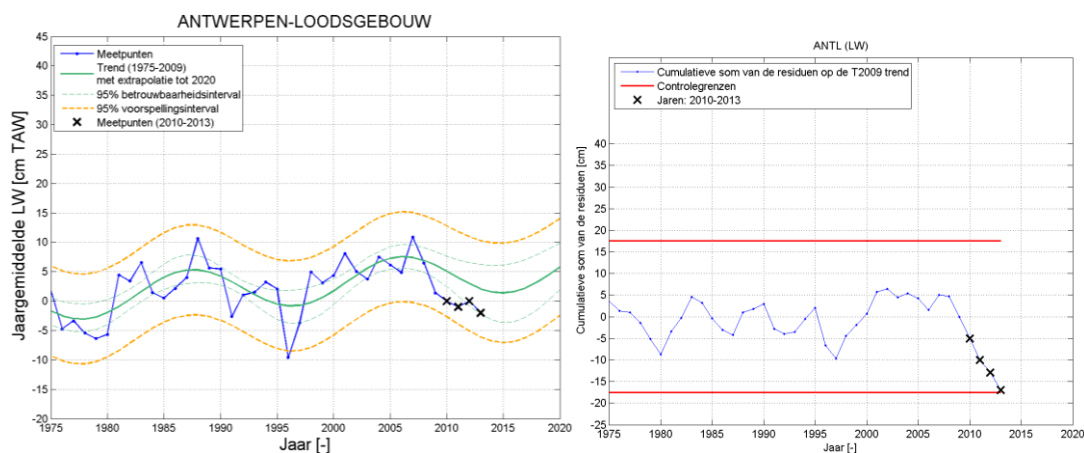
Figuur 2-15: Links: Evolutie van de jaargemiddelde laagwaterstand te Antwerpen-loodsgebouw, met T2009 trendlijn (extrapolatie tot 2020), 95 % betrouwbaarheids- en verwachtingsinterval. Rechts: Cumulatieve som van de residuen op de (geëxtrapoleerde) T2009 trend.
