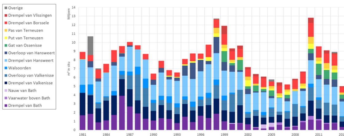
Figuur 2-3: Jaarlijks baggervolume voor alle zones in de Westerschelde tussen 1981 en 2014 (tot 01/06/2014).
