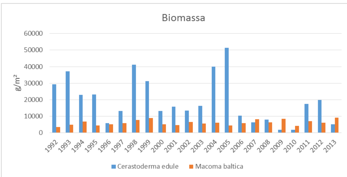
Figuur 2-49: Temporele evolutie van de biomassa van Cerastoderma edule (blauw) en Macoma baltice (oranje) in de Westerschelde tussen 1992 en 2013.
