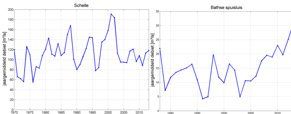
Figuur 2-11: Jaargemiddeld bovenafvoerdebiet in m 3 /s van de Schelde te Schelle (links) en de Spuisluis te Bath (rechts)
