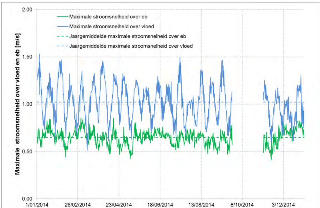
Figuur 53 - Maximale stroomsnelheid over vloed en over eb te Boei 84 (Beneden-Zeescheldebekken), bovenste meettoestel (2014)
