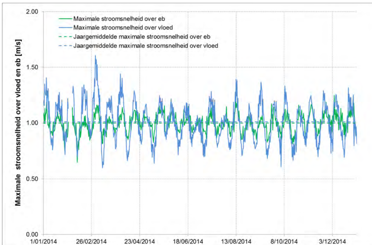
Figuur 55 - Maximale stroomsnelheid over vloed en over eb te Oosterweel (Beneden-Zeeschelde), bovenste meettoestel (2014)
