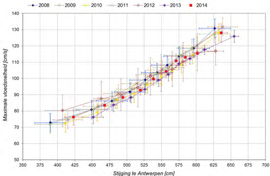
Figuur C2- 2: Maximale vloednelheid te Oosterweel (Beneden-Zeeschelde), bovenste meettoestel, versus de stijging in waterpeil te Antwerpen
