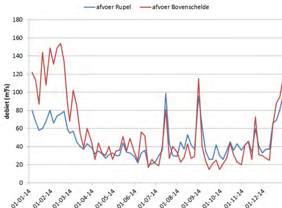
Figuur 36 - Pentadeafvoer van de Rupel en de Bovenschede opwaarts de monding van de Rupel in het jaar 2014
