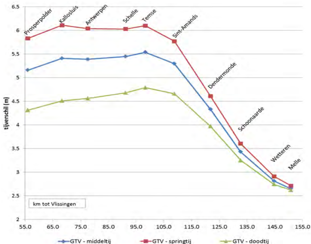
Figuur 13 - Zeeschelde: gemiddeld tijverschil (GTV) bij middeltij, springtij en doodtij in 2014 t.o.v. de afstand in km tot de monding te Vlissingen.
