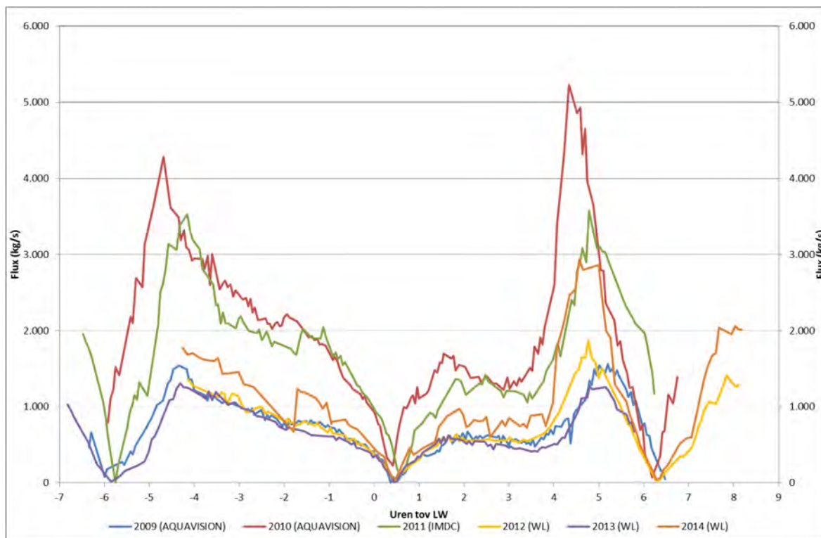
Figuur 192 - SSF tijdens de dertienuursmetingen te Oosterweel (Beneden-Zeeschelde) in 2009 t.e.m. 2014
