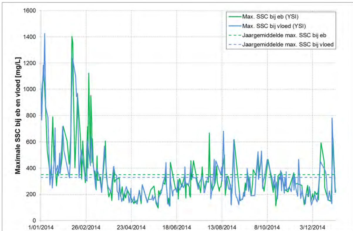
Figuur 156 - Maximale SSC bij eb en vloed te Melle (Beneden-Zeeschelde), bovenste meettoestel (2014)
