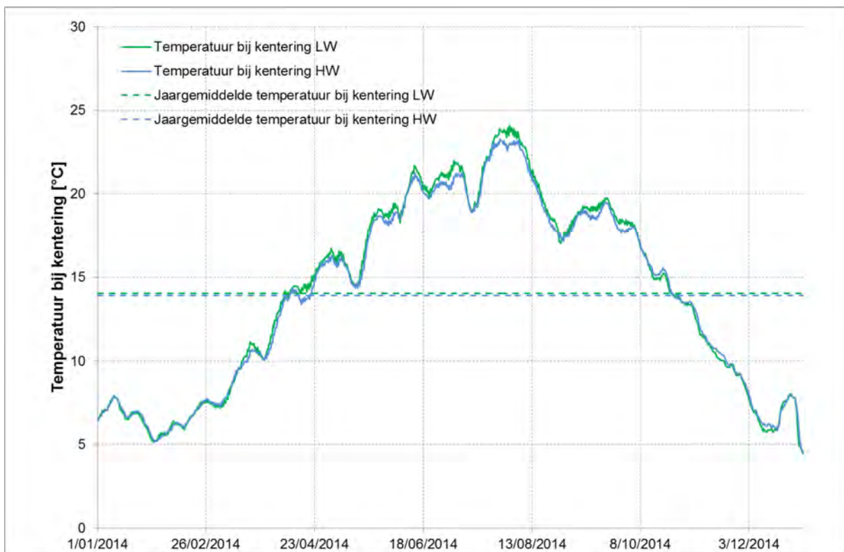
Figuur 74 - Temperatuur [°C] bij KHW en KLW te Driegoten (Boven-Zeeschelde) (2014)
