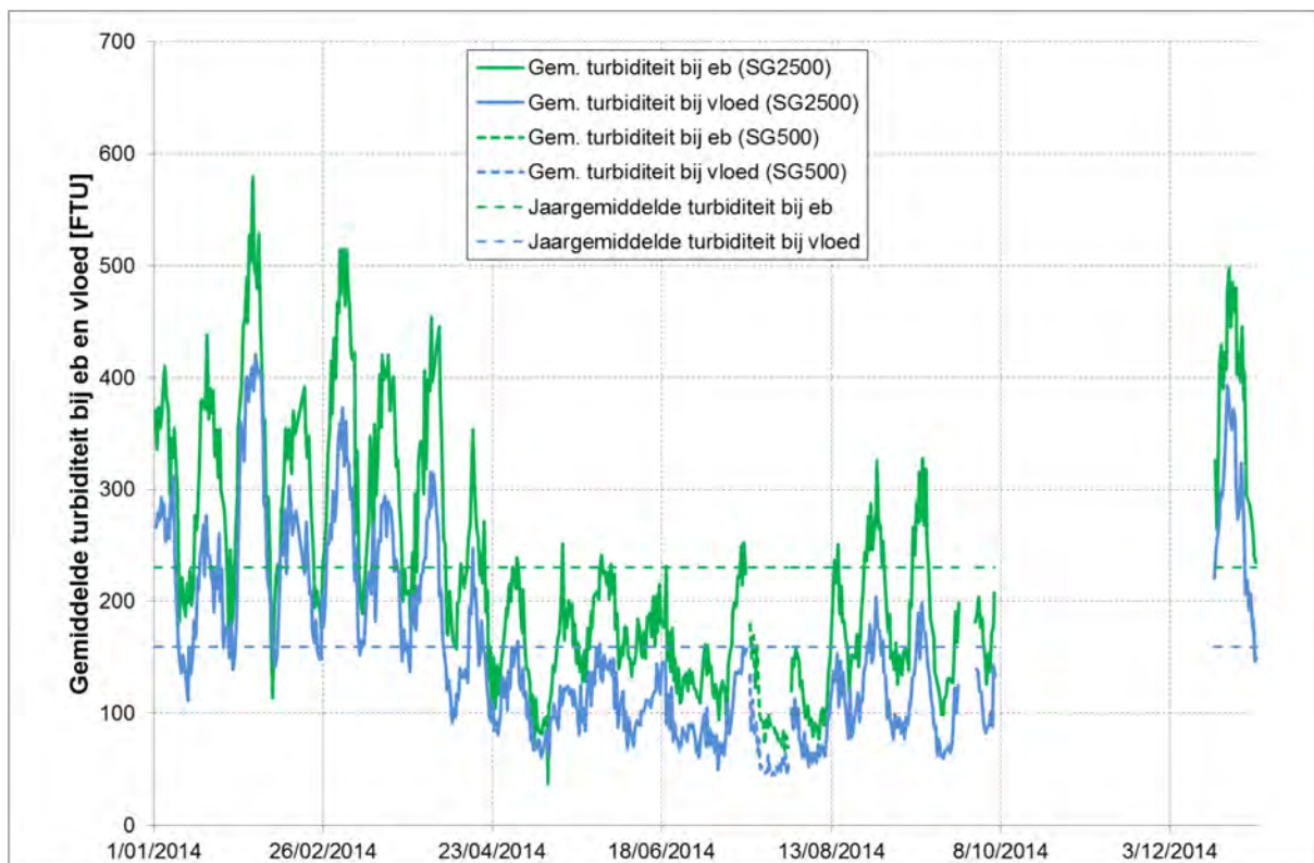
Figuur 114 - Gemiddelde turbiditeit bij eb en vloed te Boei 84 (Beneden-Zeeschelde), onderste meettoestel (2014)
