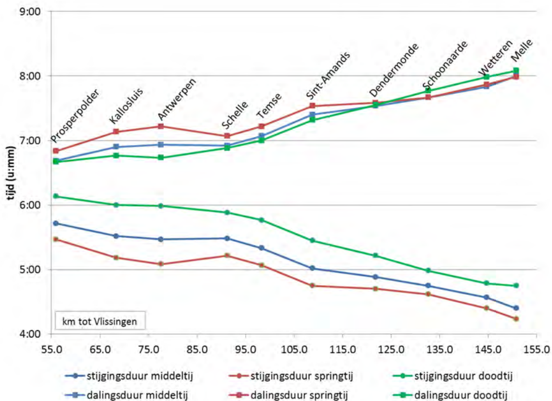
Figuur 12 - Zeeschelde: duur van stijging en daling bij middeltij, springtij en doodtij in 2014 t.o.v. de afstand in km tot de monding te Vlissingen.
