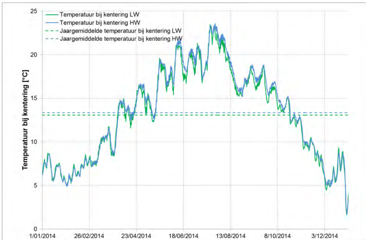
Figuur 76 - Temperatuur [°C] bij KHW en KLW te Duffel Sluis (Bededen-Nete) (2014)
