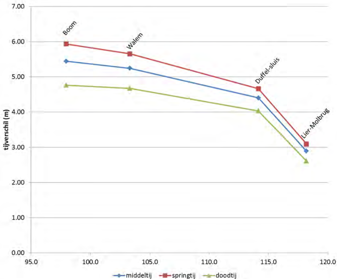
Figuur 15 - Gemiddeld tijverschil (GTV) bij middeltij, springtij en doodtij in 2014 voor de Rupel (Boom en Walem) en Beneden Nete (Duffel Sluis en Lier-Molbrug).
