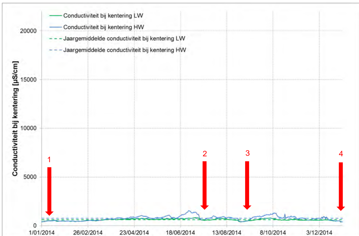
Figuur 86 - Conductiviteit bij KHW en KLW te Driegoten (Boven- Zeeschelde) (2014)
