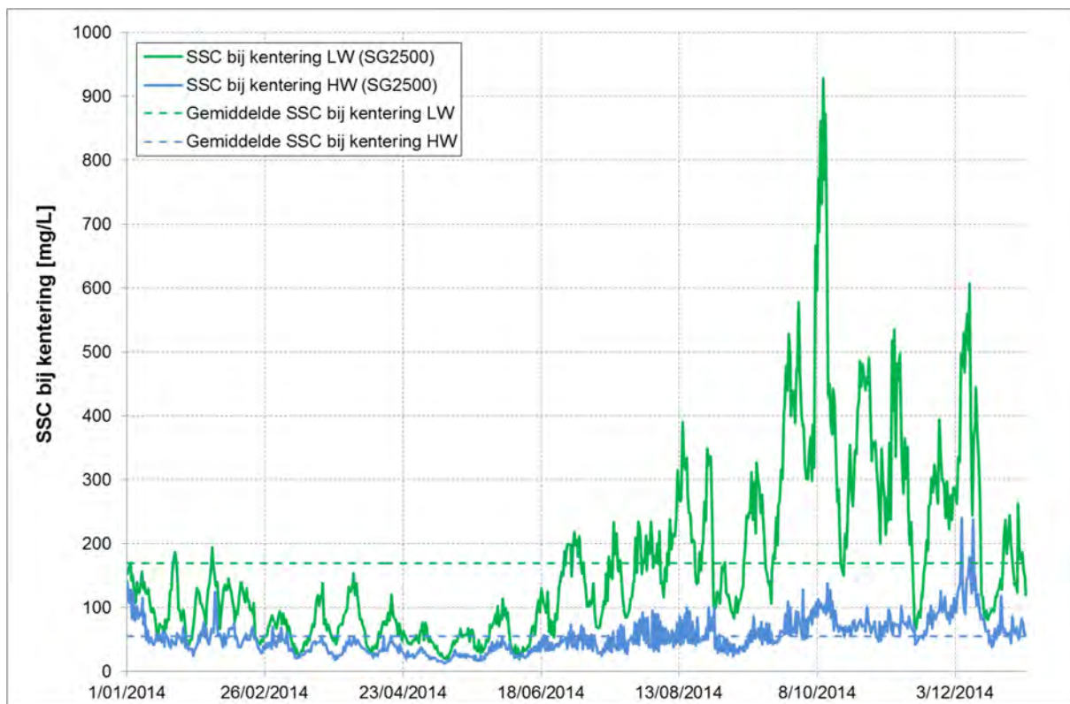
Figuur 133 - SSC bij KLW en KHW te Driegoten (Boven-Zeescheldebekken) (2014)
