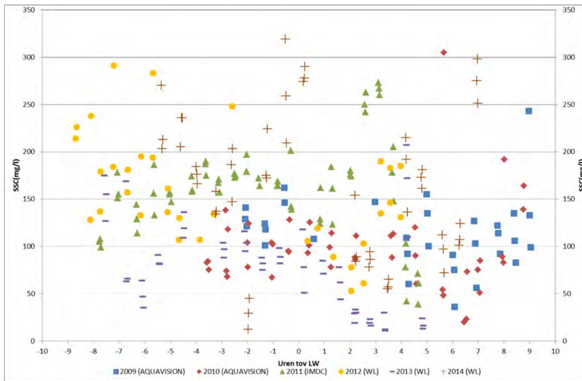
Figuur 207 - Gemeten SSC tijdens de dertienuurmetingen te Boom en Terhagen (Rupel) in 2009 t.e.m. 2014
