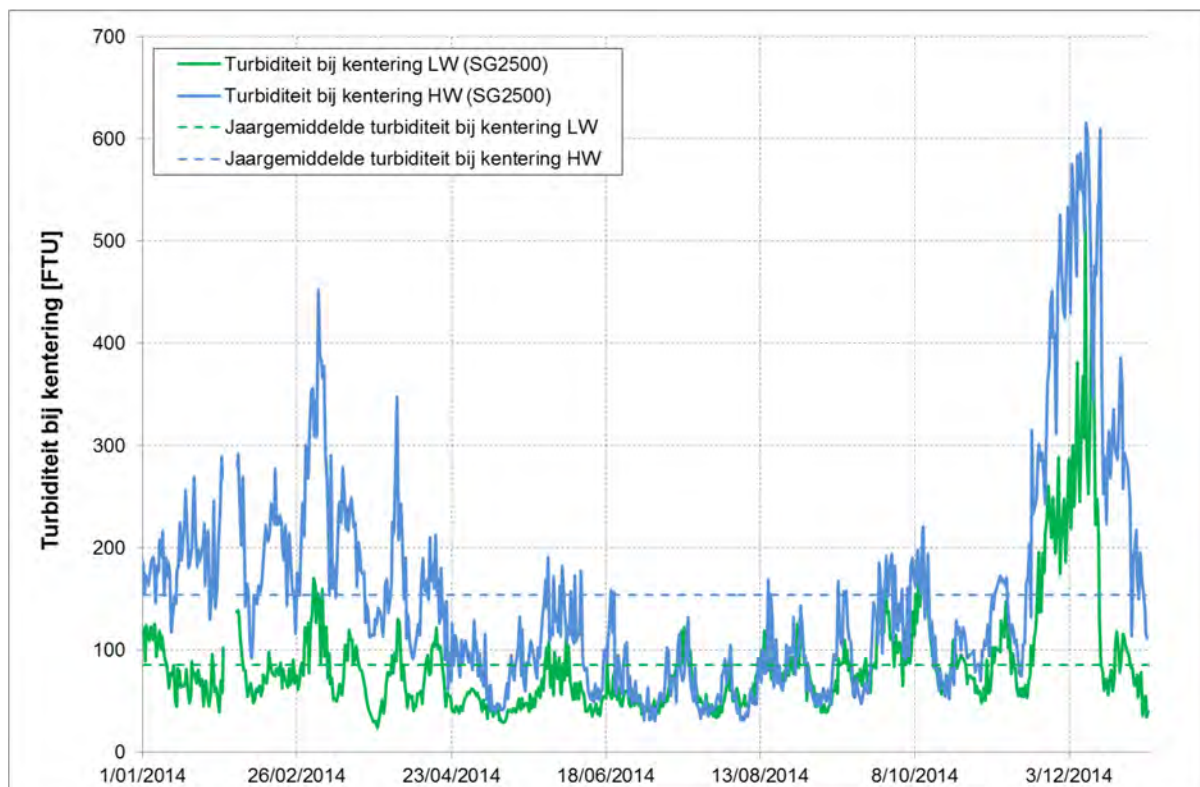
Figuur 107 - Turbiditeit bij KHW en KLW te Oosterweel (Beneden-Zeeschelde), onderste meettoestel (2014)
