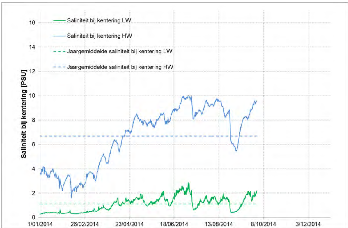
Figuur 96 - Saliniteit bij KHW en KLW te Oosterweel Boven (Beneden - Zeeschelde) (2014)
