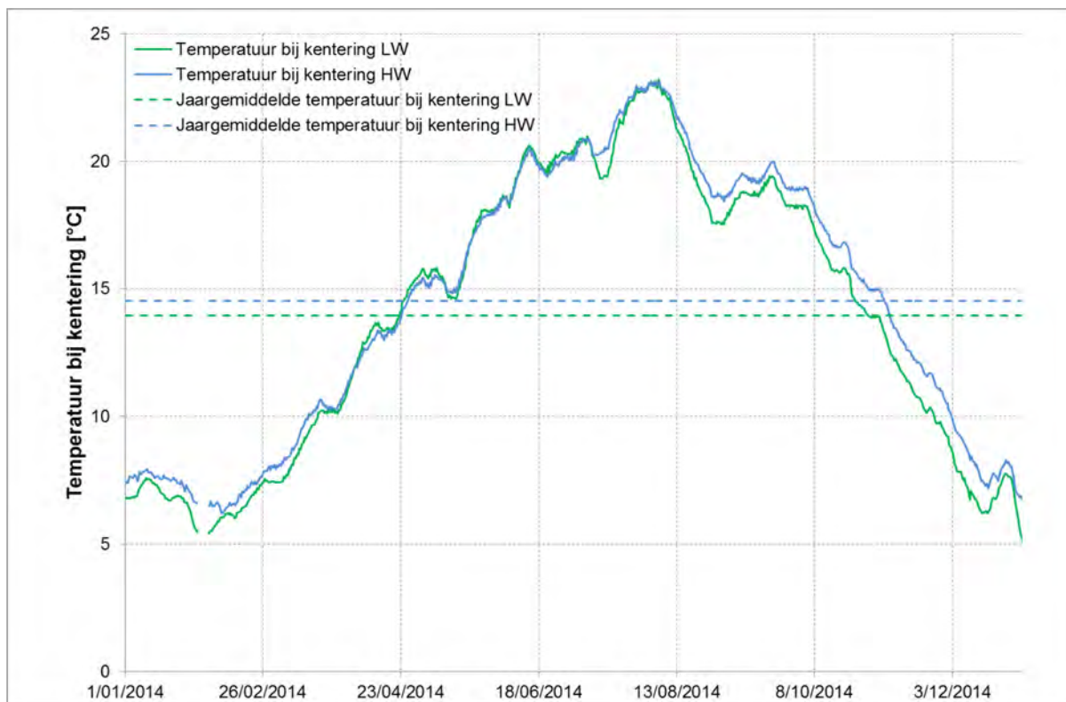
Figuur 71 - Temperatuur [°C] bij KHW en KLW te Oosterweel (Beneden-Zeeschelde), bovenste meettoestel (2014)
