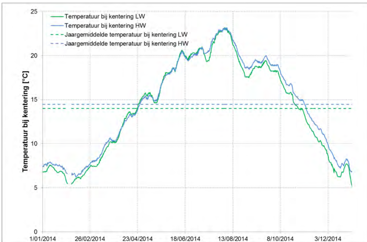
Figuur 72 - Temperatuur [°C] bij KHW en KLW te Oosterweel (Beneden-Zeeschelde), onderste meettoestel (2014)
