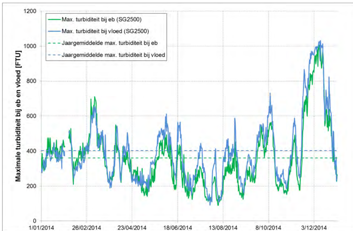
Figuur 116 - Maximale turbiditeit bij eb en vloed te Oosterweel (Beneden-Zeeschelde), onderste meettoestel (2014)
