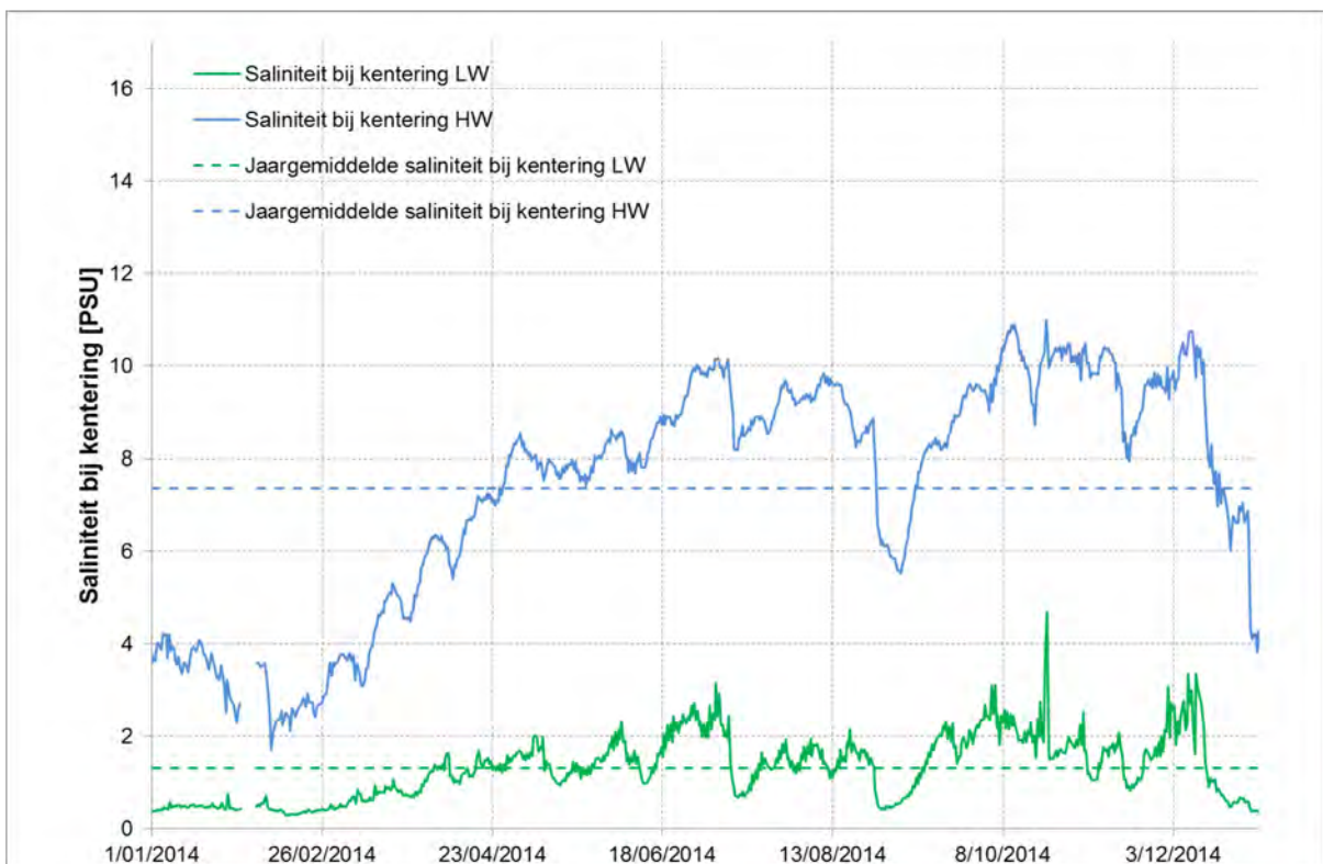
Figuur 97 - Saliniteit bij KHW en KLW te Oosterweel Onder (Beneden - Zeeschelde) (2014)
