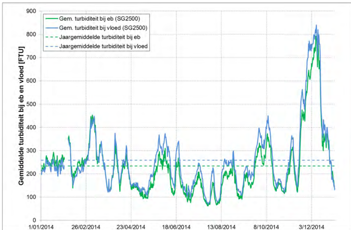
Figuur 117 - Gemiddelde turbiditeit bij eb en vloed te Oosterweel (Beneden-Zeeschelde), bovenste meettoestel (2014)
