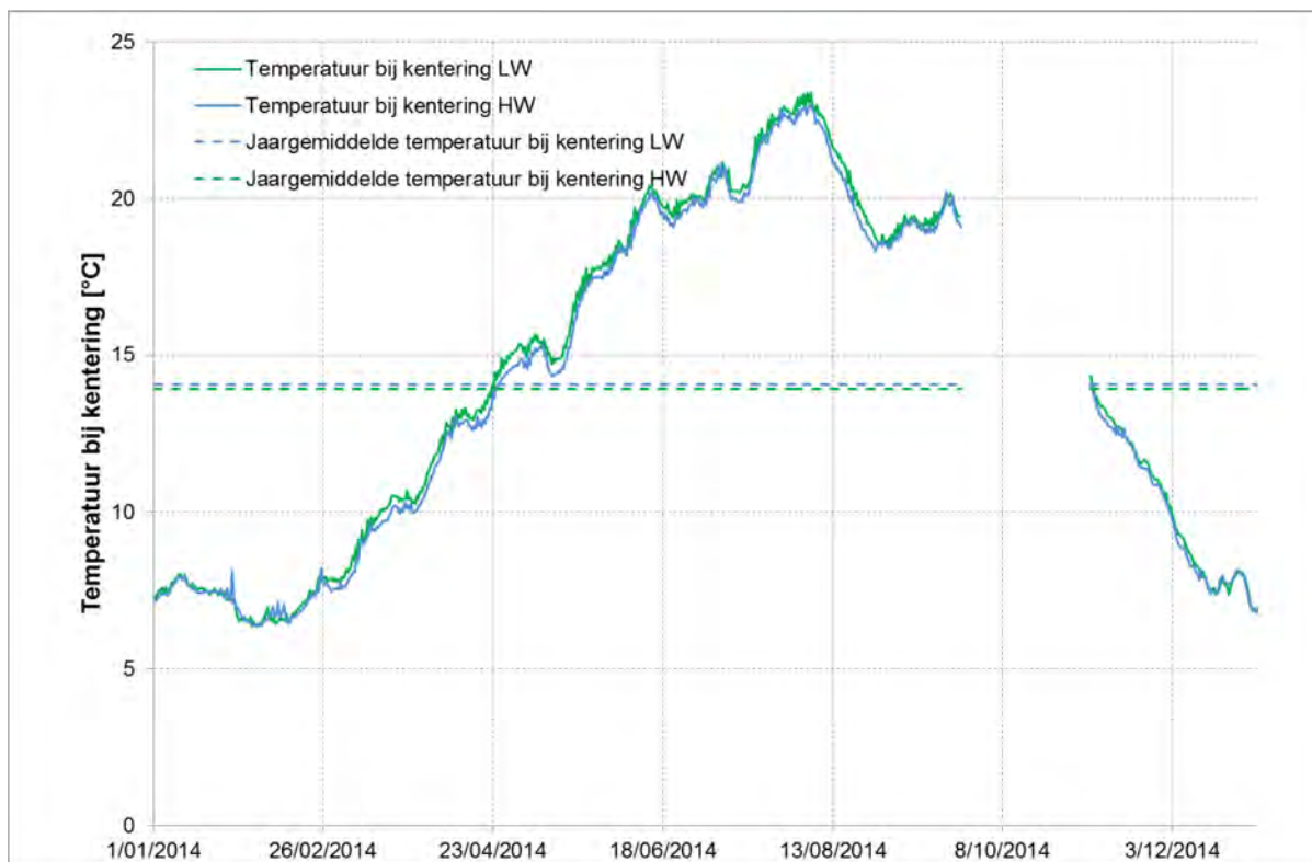
Figuur 68 – Temperatuur [°C] bij KHW en KLW te Boei 84 (Beneden-Zeescheldebekken), bovenste meettoestel (2014)
