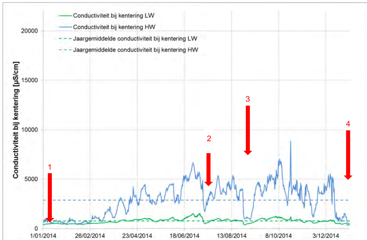
Figuur 85 - Conductiviteit bij KHW en KLW te Hemiksem (Boven - Zeeschelde) (2014)
