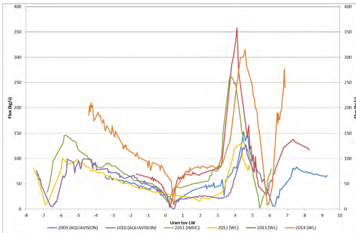
Figuur 208 - SSF tijdens de dertienuurmetingen te Boom en Terhagen (Rupel) in 2009 t.e.m. 2014
