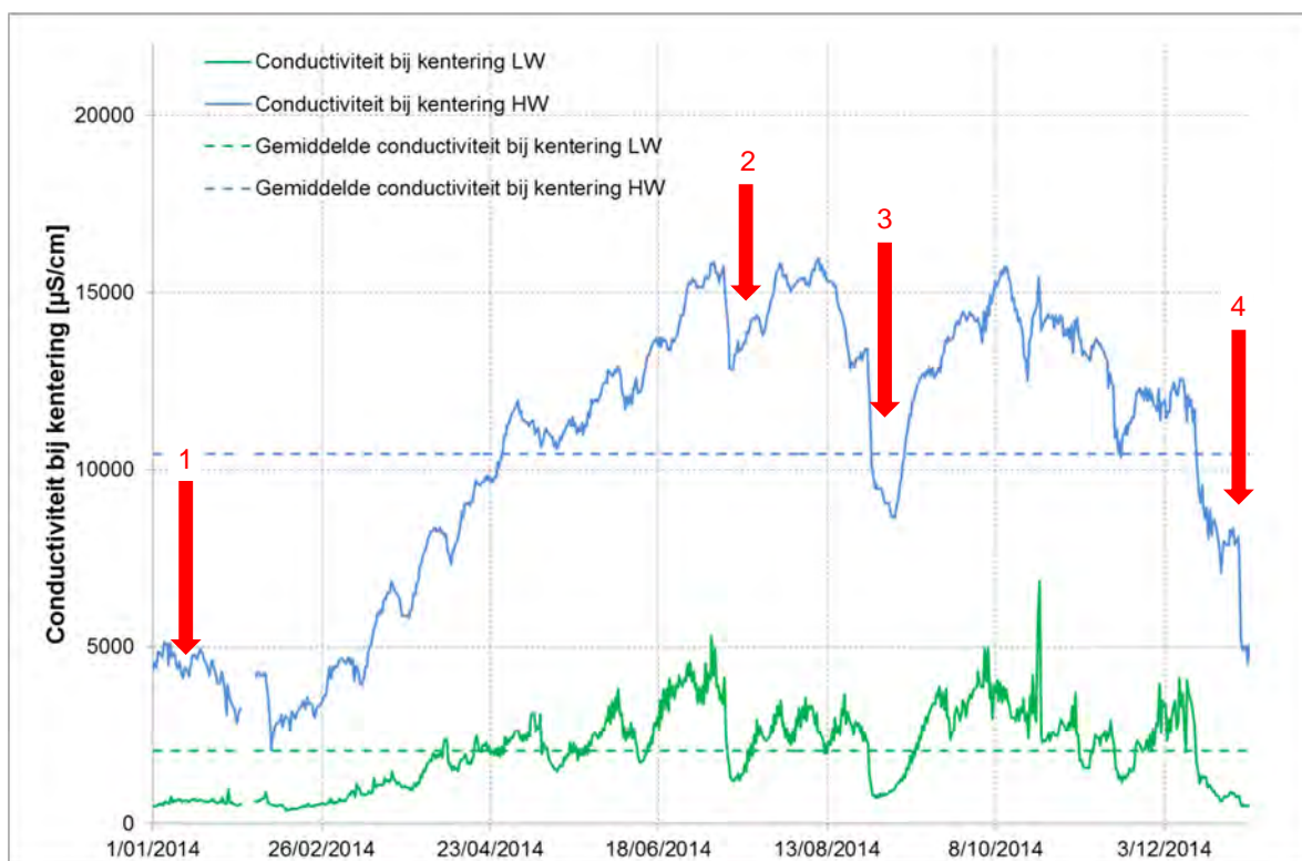
Figuur 84 - Conductiviteit bij KHW en KLW te Oosterweel (Beneden- Zeeschelde), onderste meettoestel (2014)
