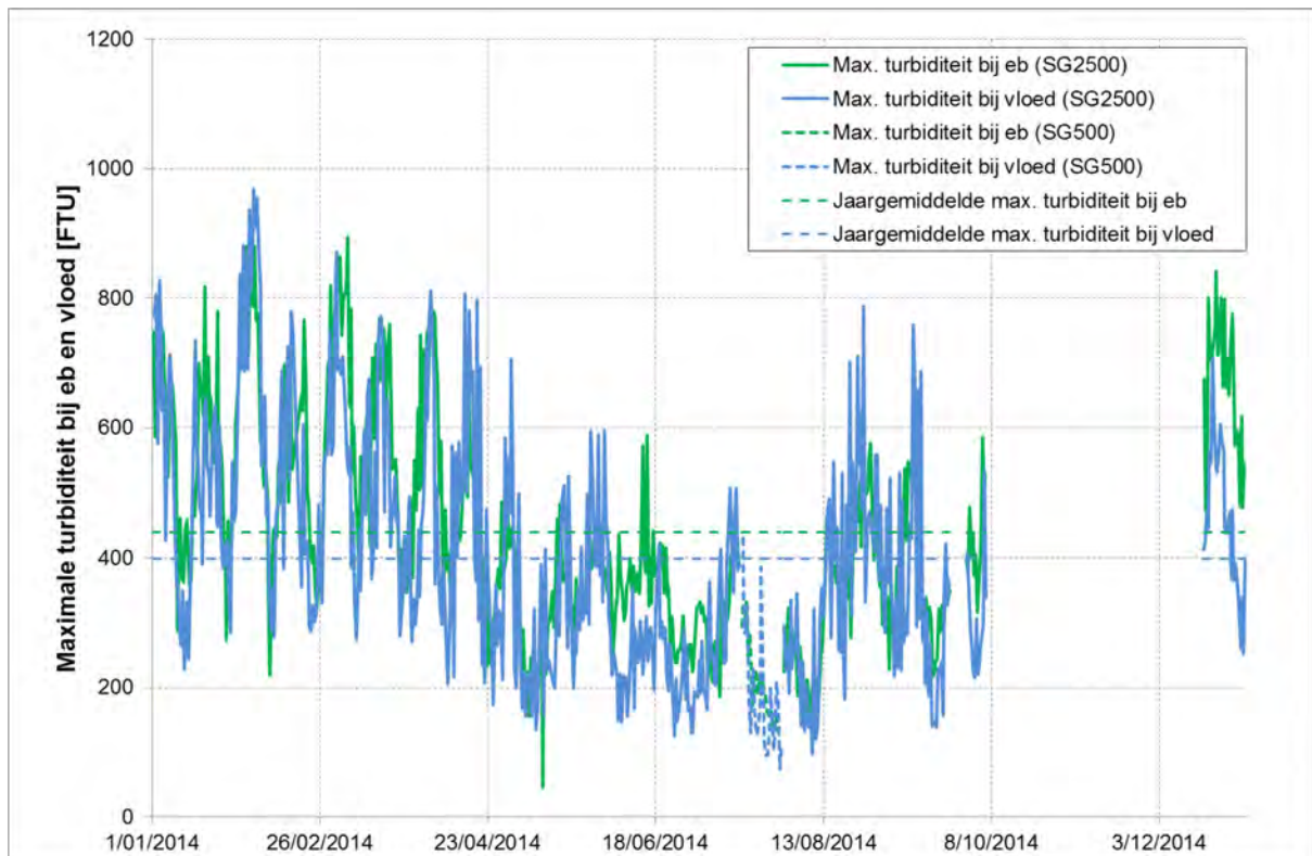
Figuur 112 - Maximale turbiditeit bij eb en vloed te Boei 84 (Beneden-Zeescheldebekken), onderste meettoestel (2014)
