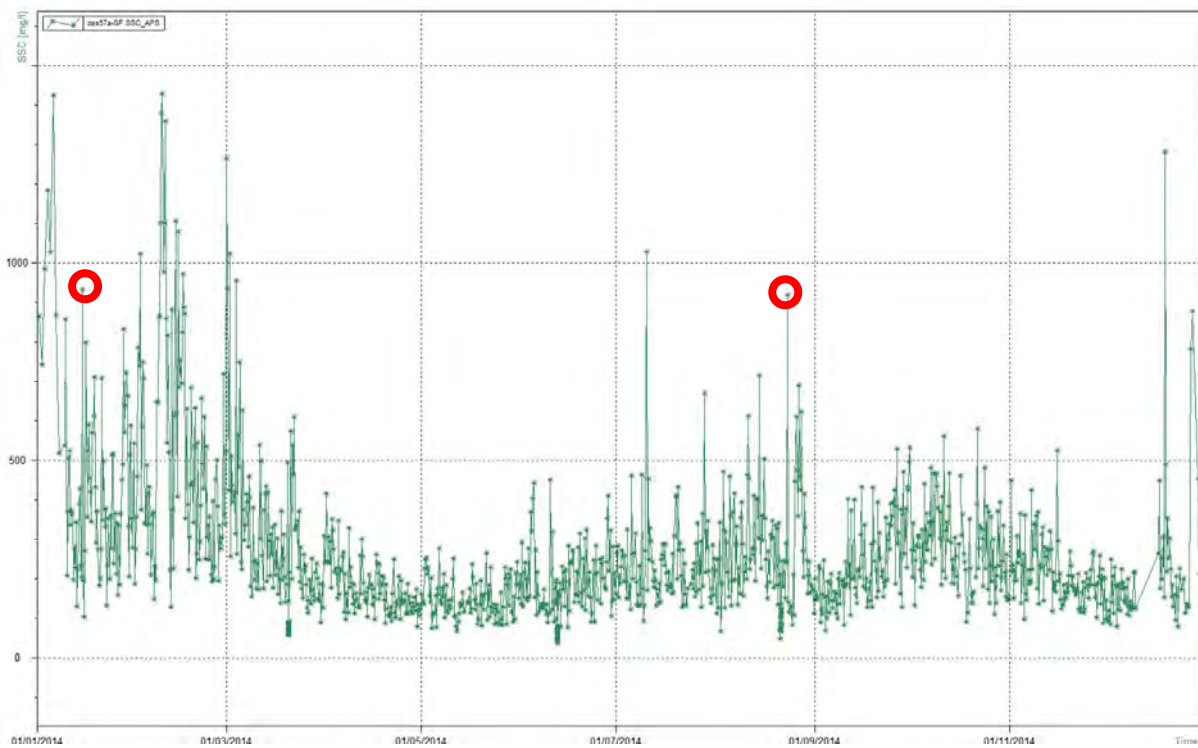
Figuur 147 - SSC (gemeten m.b.v. automatische stalname) te Melle (Boven-Zeeschelde)
