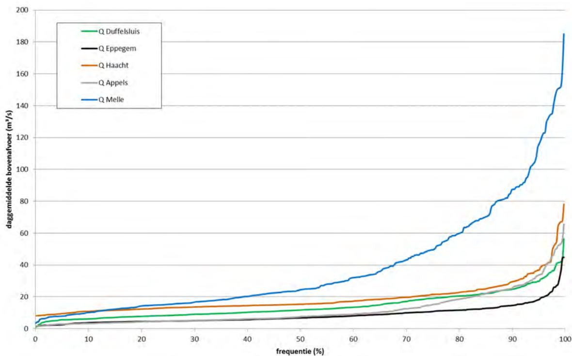
Figuur 35 - Zeescheldebekken: sortering naar grootte van de daggemiddelde bovendebielen aan de meetraaien in het jaar 2014
