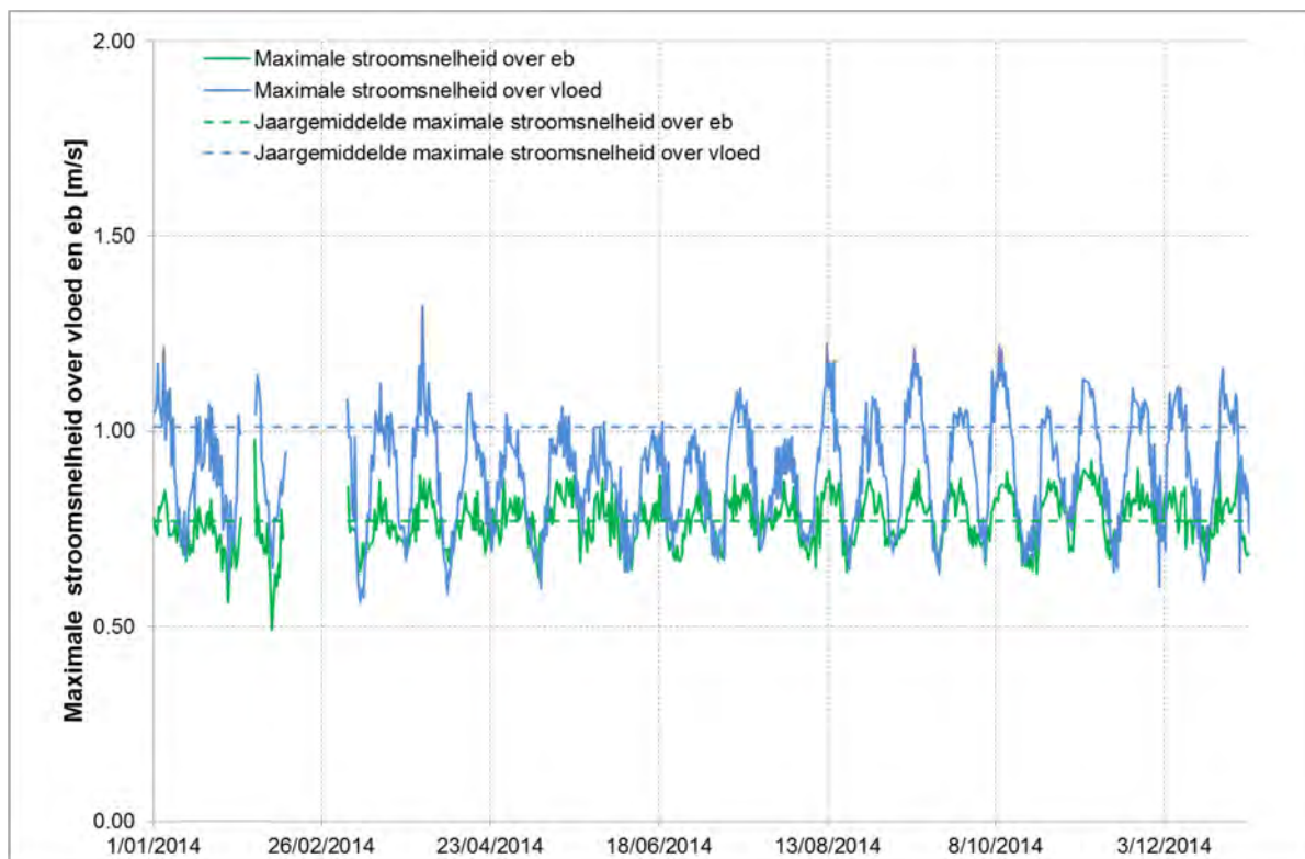
Figuur 56 - Maximale stroomsnelheid over vloed en over eb te Oosterweel (Beneden-Zeeschelde), onderste meettoestel (2014)
