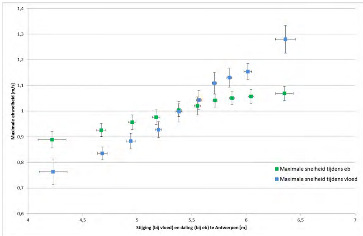
Figuur 65 - Maximale ebsnelheid en maximale vloodsnelheid te Oosterweel (Beneden-Zeeschelde), onderste meettoestel, versus de daling, respectievelijk de stijging, in waterpeil te Antwerpen (2014)
