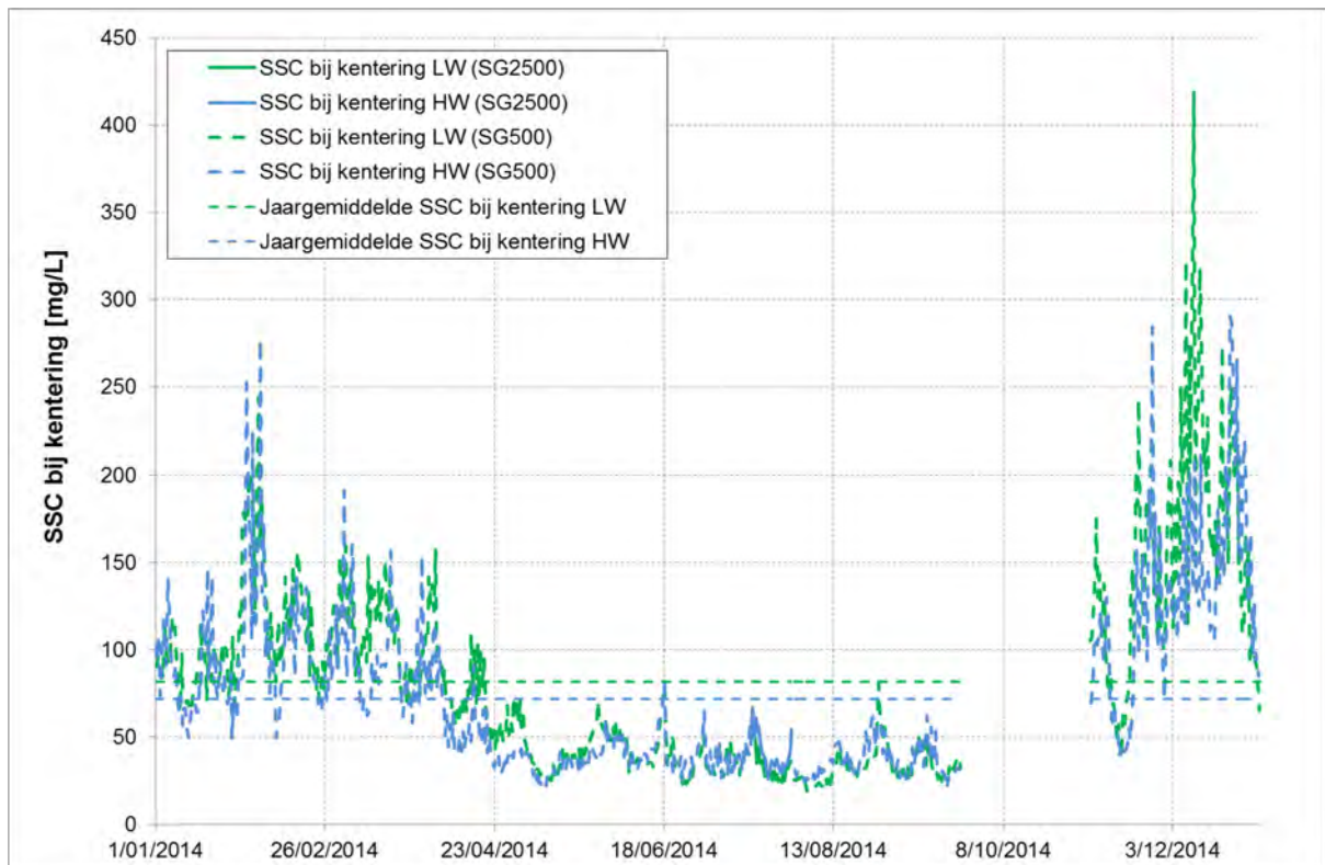
Figuur 129 - SSC bij K LW en K HW te Boei 84 (Beneden -Zeeschelde), bovenste meettoestel (2014)
