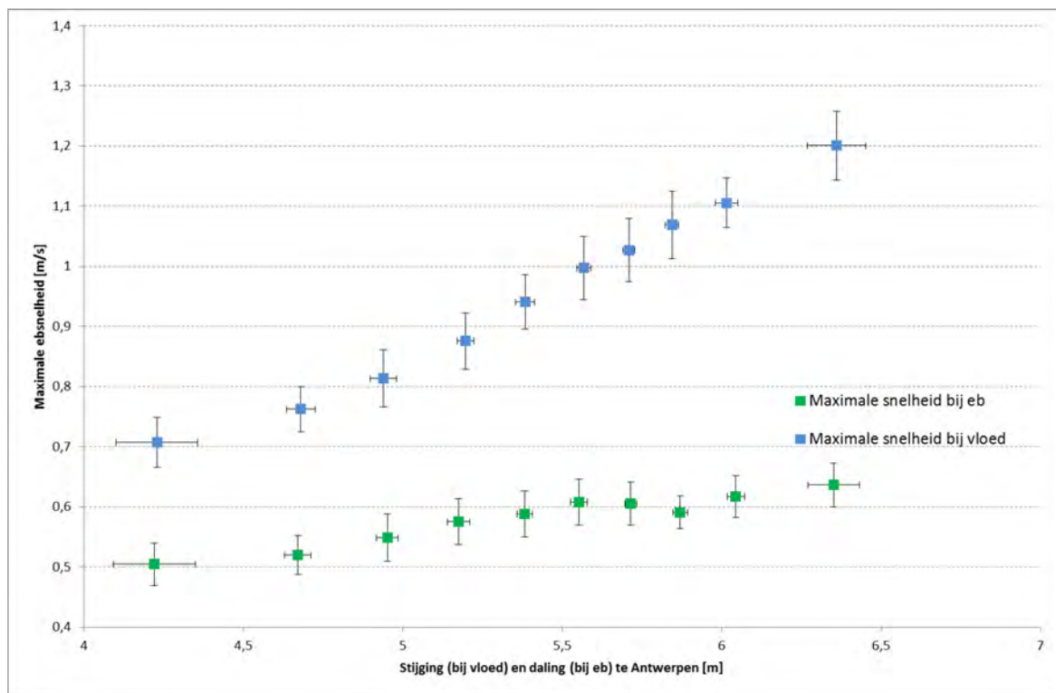
Figuur 63 - Maximale ebsnelheid en maximale vloedsnelheid te Boei 84 (Beneden-Zeeschelde), onderste meettoestel, versus de daling, respectievelijk de stijging, in waterpeil te Antwerpen (2014)
