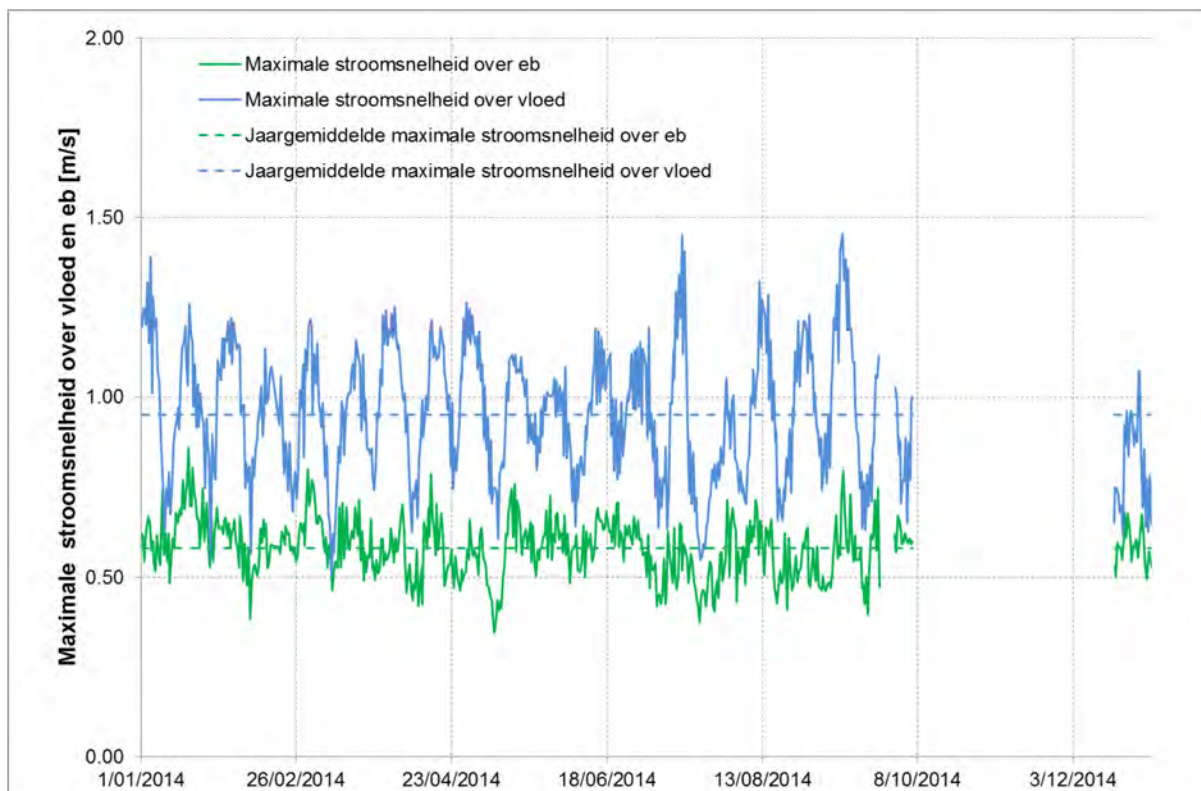
Figuur 54 - Maximale stroomsnelheid over vloed en over eb te Boei 84 (Beneden-Zeeschelde), onderste meettoestel (2014)
