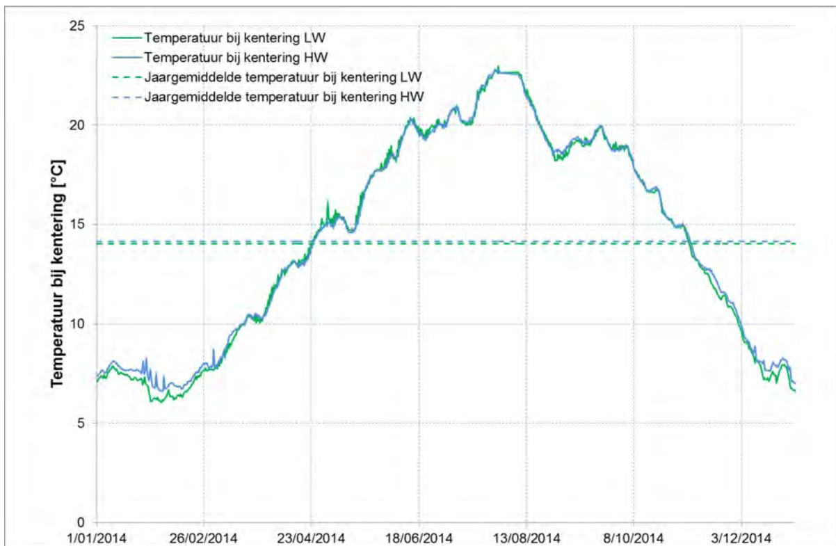
Figuur 70 - Temperatuur [°C] bij KHW en KLW te Liefkenshoek (Beneden-Zeeschelde) (2014)
