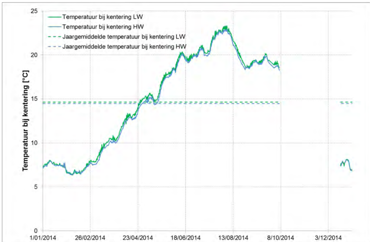
Figuur 69 - Temperatuur [°C] bij KHW en KLW te Boei 84 (Beneden-Zeeschelde), onderste meettoestel (2014)
