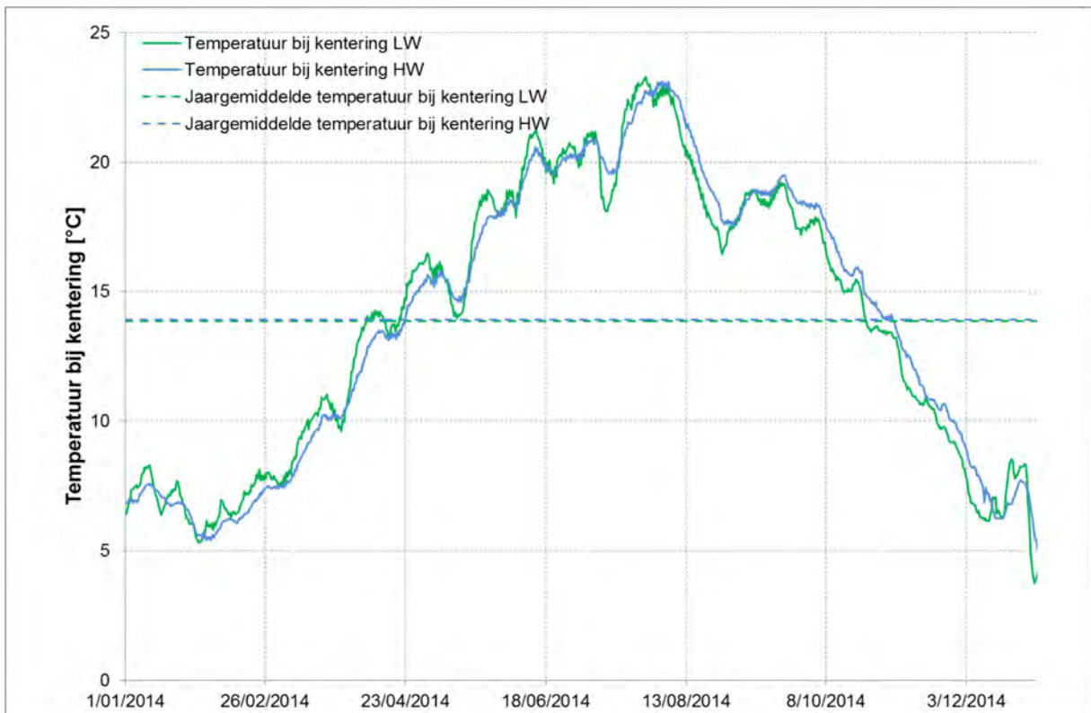
Figuur 73 - Temperatuur [°C] bij KHW en KLW te Hemiksem (Boven-Zeeschelde) (2014)
