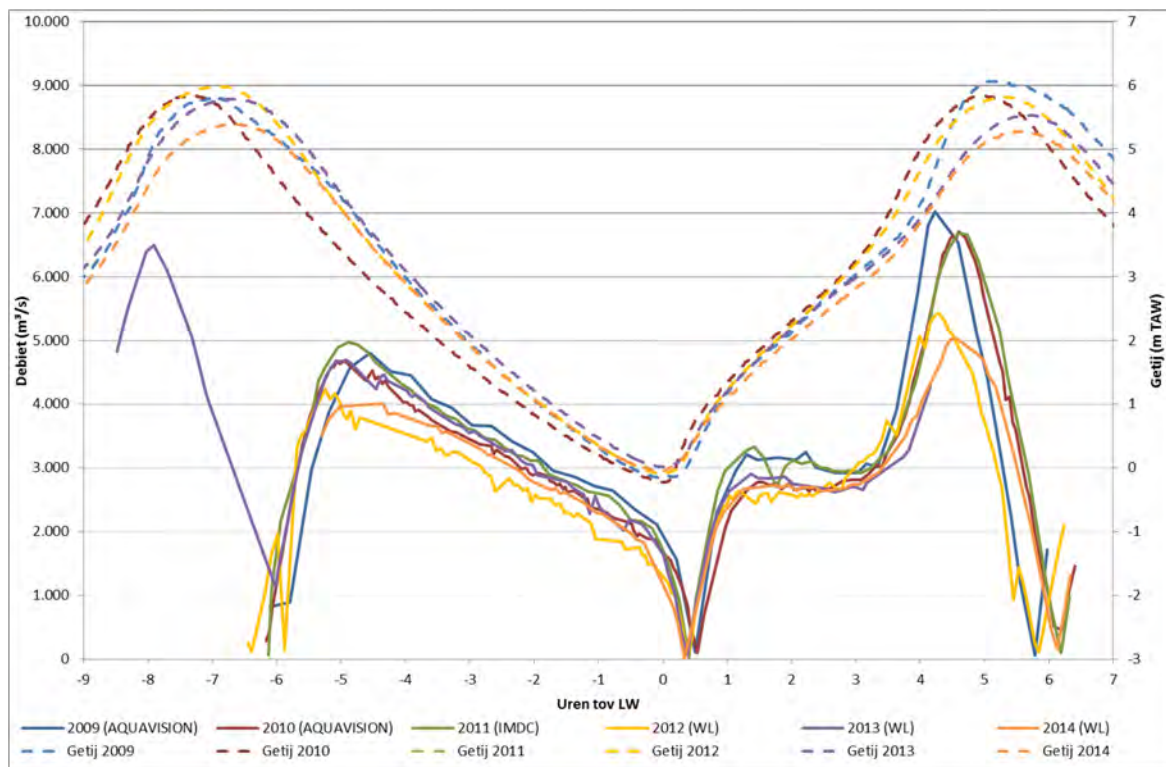
Figuur 194 - Debiet en getij tijdens de dertienuursmetingen te Kruikebe (Beneden-Zeeschelde) in 2009 t.e.m. 2014
