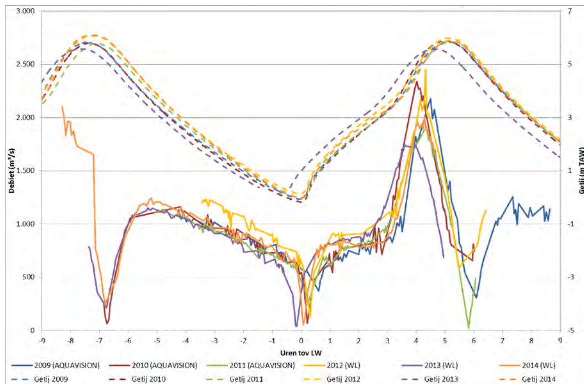
Figuur 198 - Debiet en getij tijdens de dertienuursmetingen te Driegoten (Boven-Zeeschelde) in 2009 t.e.m. 2014
