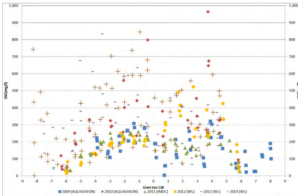
Figuur 199 - Gemeten SSC tijdens de dertienuursmetingen te Driegoten (Boven-Zeeschelde) in 2009 t.e.m. 2014
