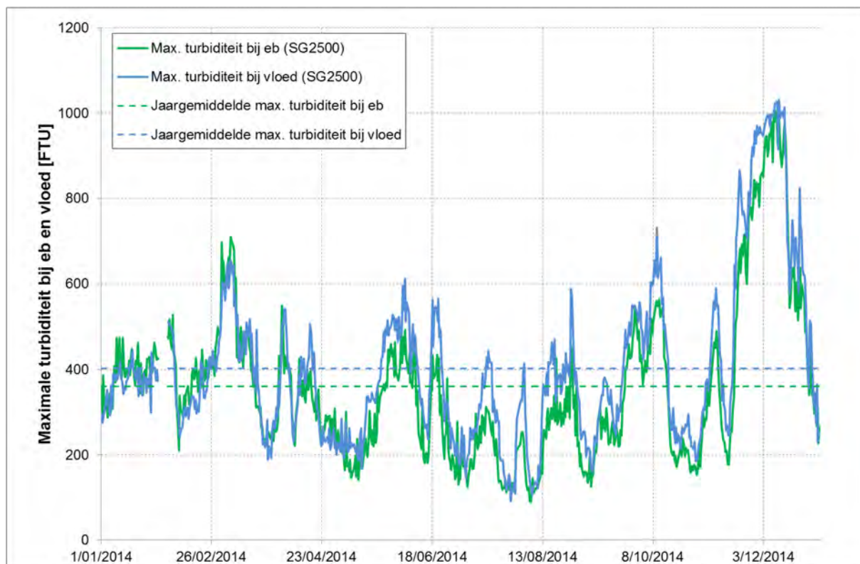
Figuur 115 - Maximale turbiditeit bij eb en vloed te Oosterweel (Beneden-Zeeschelde), bovenste meettoestel (2014)
