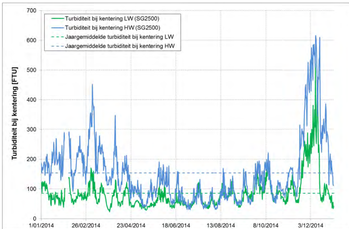
Figuur 106 - Turbiditeit bij KHW en KLW te Oosterweel (Beneden-Zeeschelde), bovenste meettoestel (2014)
