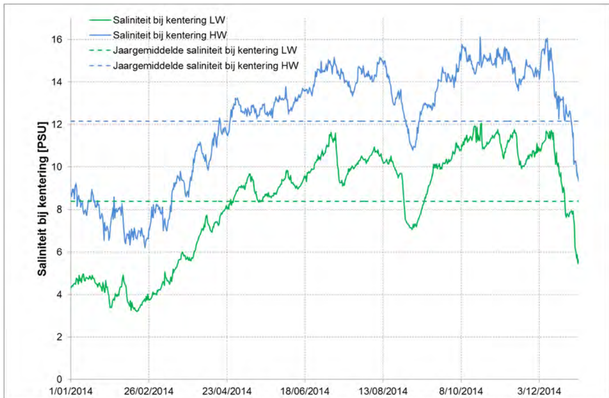
Figuur 92 - Saliniteit bij KHW en KLW te Prosperpolder (Beneden - Zeeschelde) (2014)
