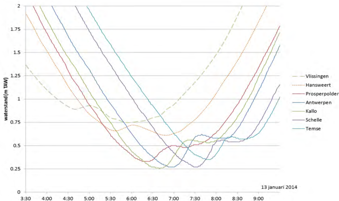
Figuur 19 - Speciaal tij op 13 januari 2014. Meetposten te Vlissingen, Hansweert, Prosperpolder, Kallo, Antwerpen, Schelle en Temse (tijden in UTC).
