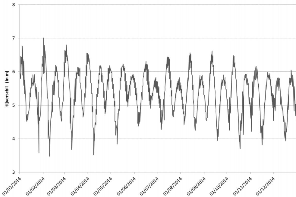
Figuur 2 - Verloop van tjiverschil geobserveerd in Antwerpen (Beneden Zeeschelde) in 2014.
