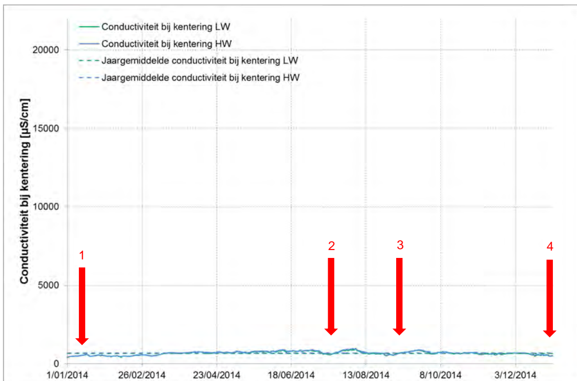
Figuur 87 - Conductiviteit bij KHW en KLW te Melle (Boven- Zeeschelde) (2014)
