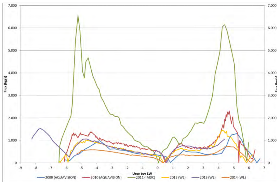
Figuur 196 - SSF tijdens de dertienuursmetingen te Kruibeke (Beneden-Zeeschelde) in 2009 t.e.m. 2014
