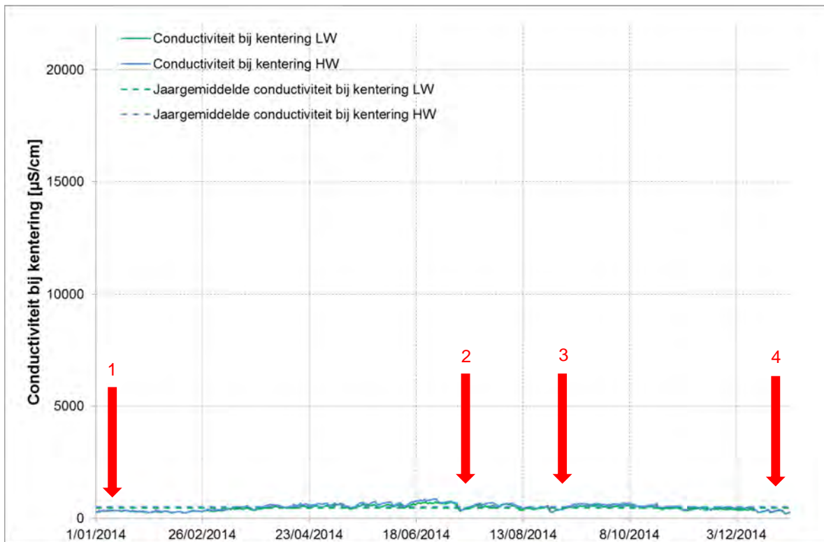
Figuur 88 - Conductiviteit bij KHW en KLW te Duffel Sluis (Beneden - Nete) (2014)
