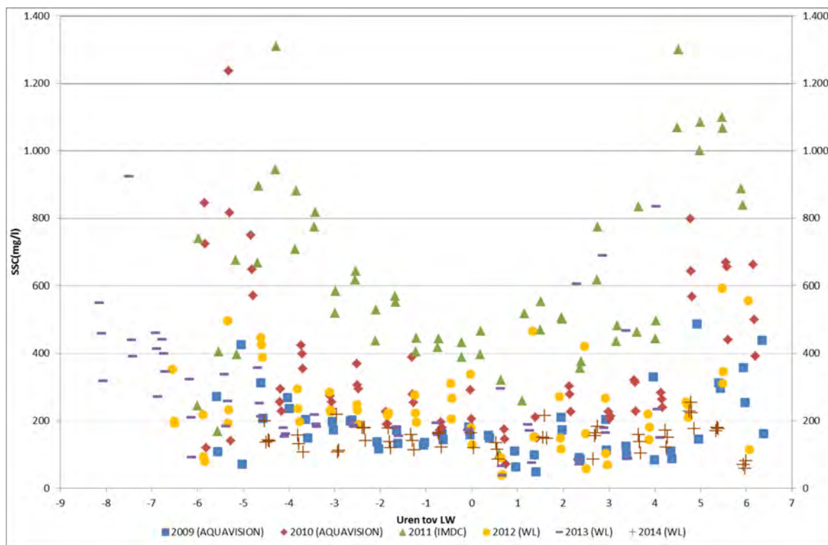
Figuur 195 - Gemeten SSC tijdens de dertienuursmetingen te Kruikebe (Beneden-Zeeschelde) in 2009 t.e.m. 2014
