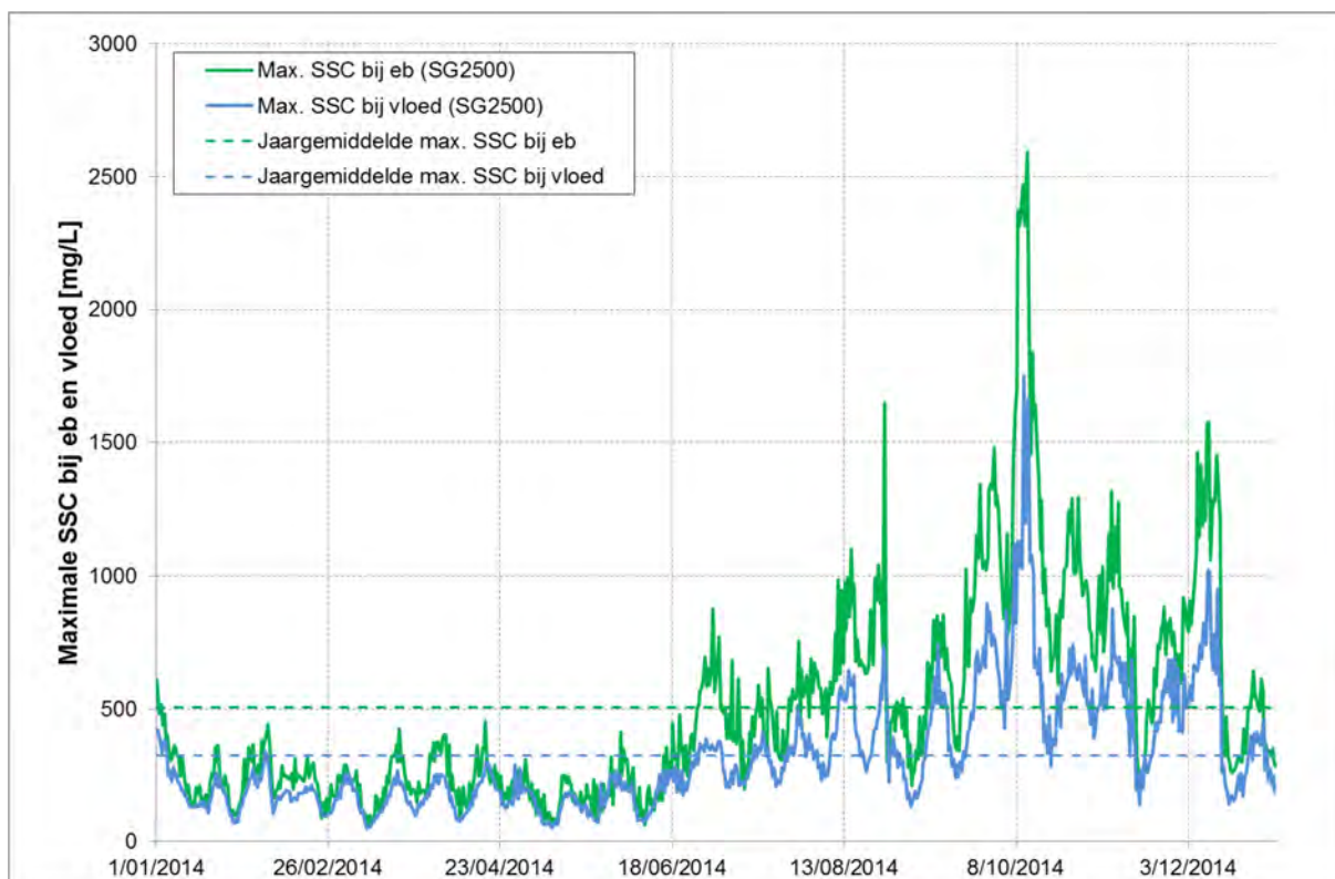
Figuur 142 - Maximale SSC bij eb en vloed te Driegoten (Boven-Zeeschelde) (2014)
