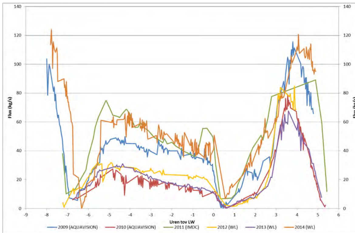
Figuur 204 - SSF tijdens de dertienuursmetingen te Schoonaarde (Boven-Zeeschelde) in 2009 t.e.m. 2014
