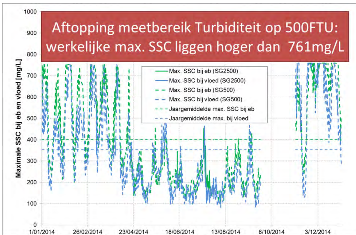
Figuur 134 - Maximale SSC bij eb en vloed te Boei 84 (Beneden-Zeescheldebekken), bovenste meettoestel (2014)
