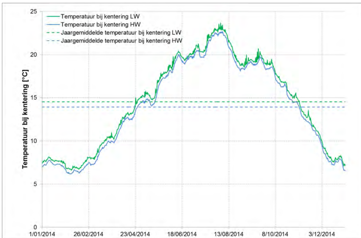
Figuur 67 - Temperatuur [°C] bij KHW en KLW te Prosperpolder (Beneden-Zeescheldebekken) (2014)
