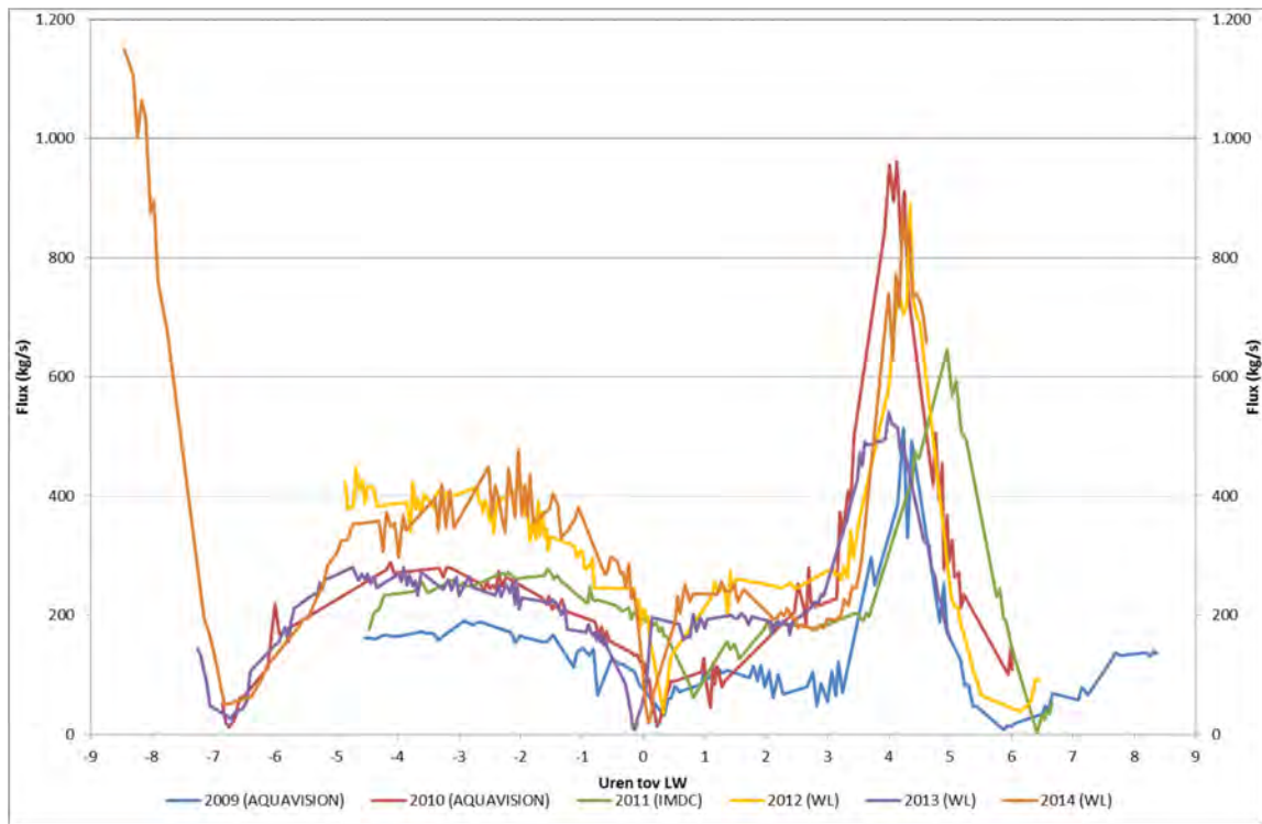
Figuur 200 - SSF tijdens de dertienuursmetingen te Driegoten (Boven-Zeeschelde) in 2009 t.e.m. 2014
