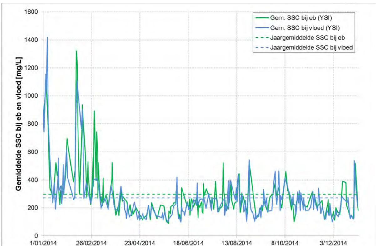
Figuur 157 - Gemiddelde SSC bij eb en vloed te Melle (Beneden-Zeeschelde), bovenste meettoestel (2014)
