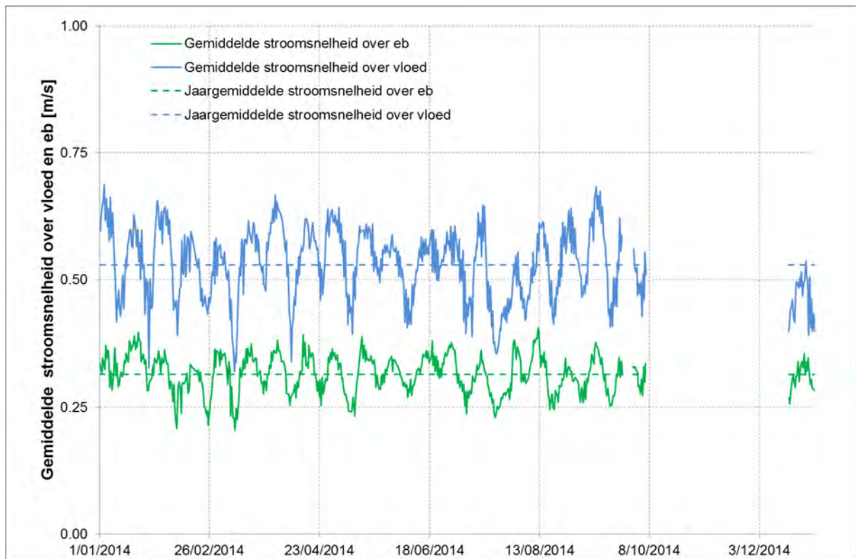
Figuur 49 - Gemiddelde stroomsnelheid over vloed en over eb te Boei 84 (Beneden-Zeeschelde), onderste meettoestel (2014)
