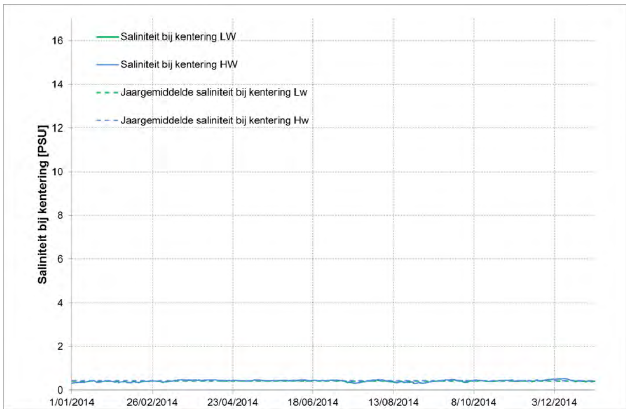
Figuur 100 - Saliniteit bij KHW en KWL te Melle (Boven - Zeeschelde) (2014)
