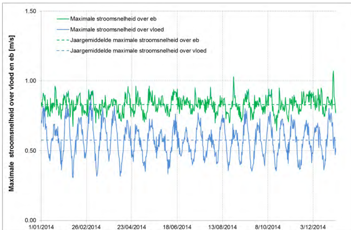
Figuur 57 - Maximale stroomsnelheid over vloed en over eb te Driegoten (Boven-Zeeschelde) (2014)
