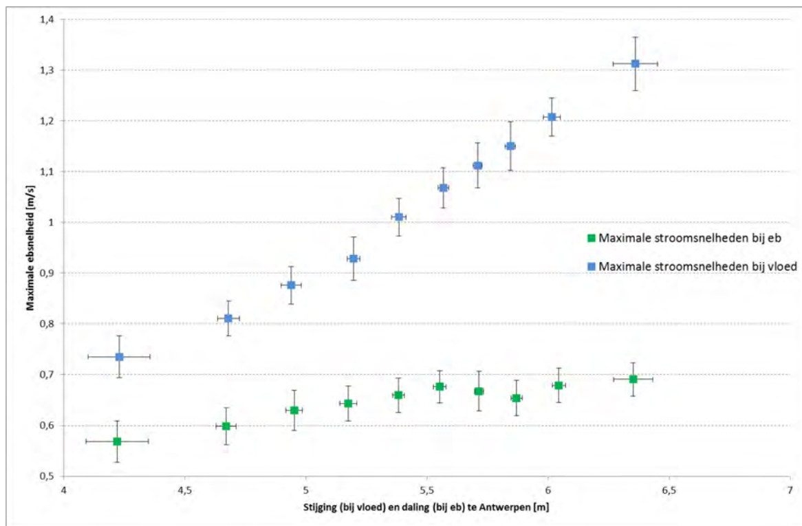
Figuur 62 - Maximale ebsnelheid en maximale vloedsnelheid te Boei 84 (Beneden-Zeeschelde), bovenste meettoestel, versus de daling, respectievelijk de stijging, in waterpeil te Antwerpen (2014)
