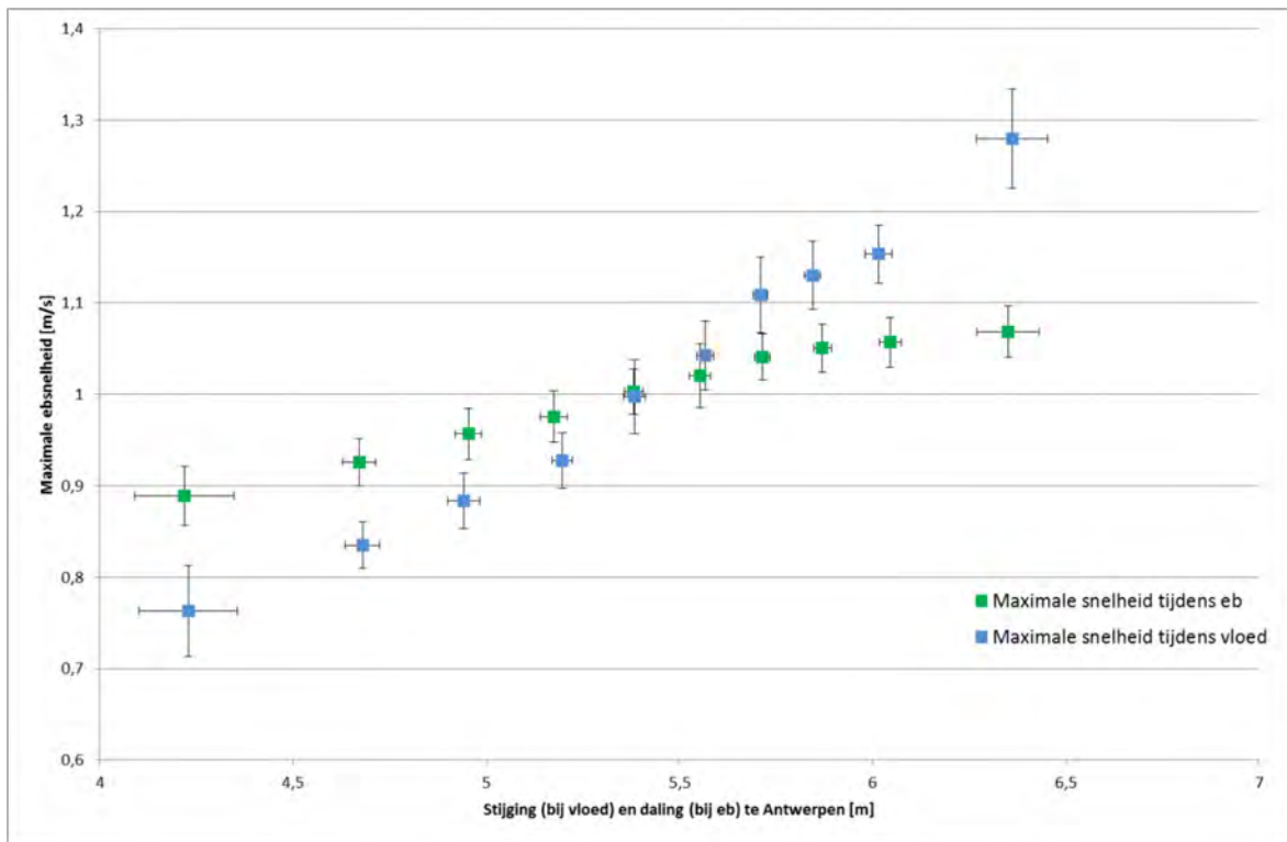
Figuur 64 - Maximale ebsnelheid en maximale vloodsnelheid te Oosterweel (Beneden-Zeeschelde), bovenste meettoestel, versus de daling, respectievelijk de stijging, in waterpeil te Antwerpen (2014)
