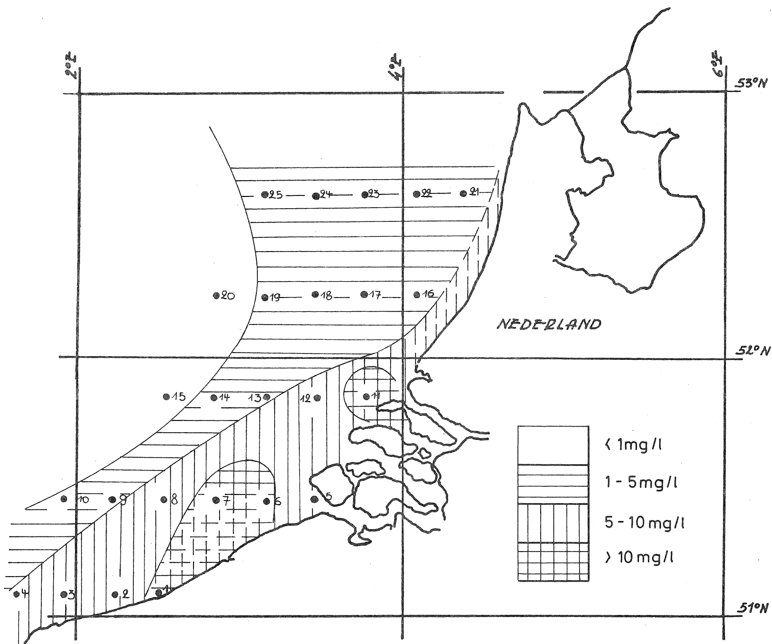
fig. 22. Maximale waargenomen suspensiegehalten
