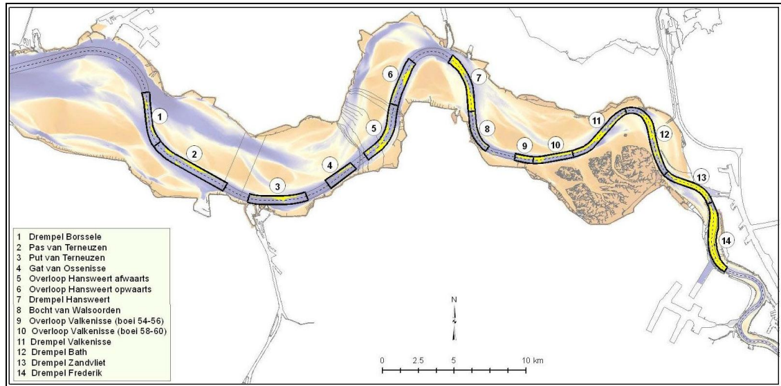
Figuur 30 Drempels in het Schelde estuarium.
