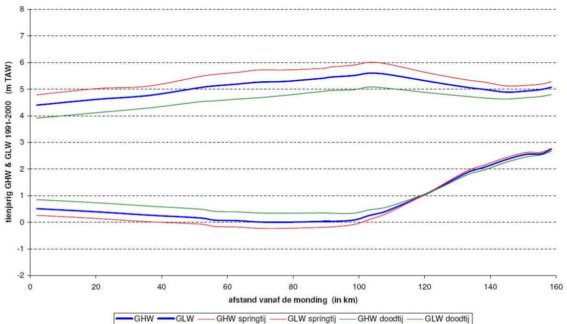
Figuur 3 Meetkundige plaats van de hoog- en laagwaters voor de periode 1991-2000 van de Schelde (bron: ir. E. Taverniers).
