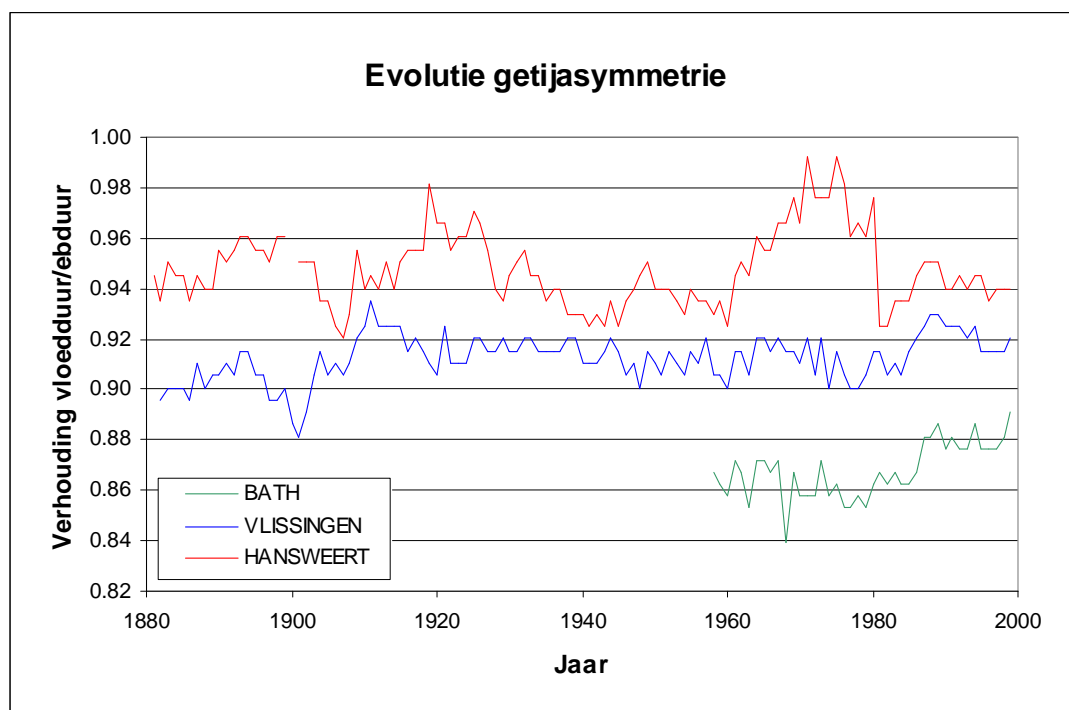
Figuur 10 Evolutie van getijasymmetrie op basis van waterstanden in verschillende stations langs het Schelde-estuarium (bron: RIKZ). Ebduur is bepaald als de tijdsduur van hoogwater naar laagwater. Vloedduur is de periode van laagwater tot hoogwater.
