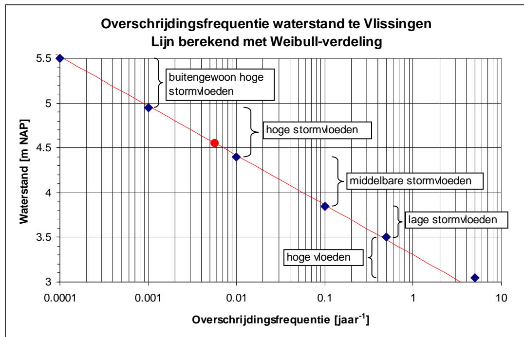
Figuur 14a Overschrijdingsfrequenties van waterstanden te Vlissingen (gebaseerd op gegevens in RIKZ, 2004). Datapunten (♦) volgens Tabel 1.
